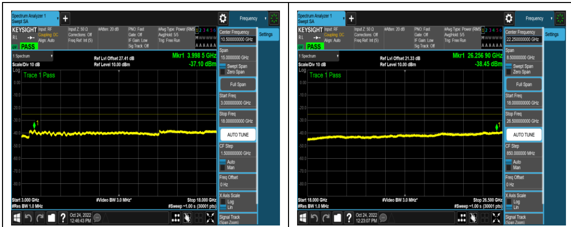
1-N41-PC3-30-70-H-4-N/A-DFT-QPSK-Edge _1RB_Left-1@0-3000-18000-Ant1-3690.50-- 37.10--25-PASS
