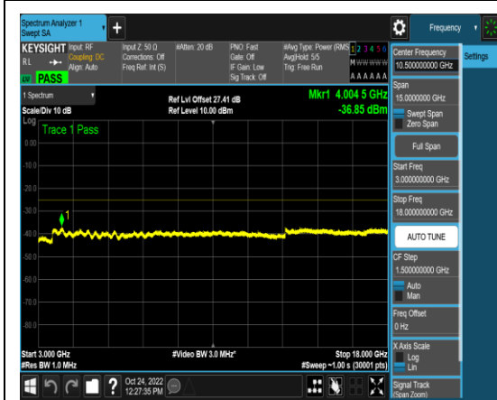
1-N41-PC3-30-80-L-4-N/A-DFT-QPSK-Edge _1RB_Left-1@0-3000-18000-Ant1-4027.50-- 36.85--25-PASS
