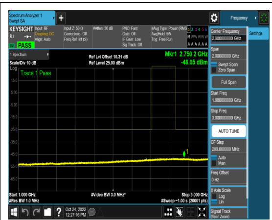
1-N41-PC3-30-80-L-4-N/A-DFT-QPSK-Edge _1RB_Left-1@0-1000-3000-Ant1-2682.90--4 8.05--25-PASS
