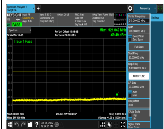
1-N41-PC3-30-70-H-16-N/A-CP-QPSK-Edge _1RB_Left-1@0-30-1000-Ant1-916.19--69.49 --35-PASS
