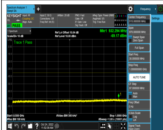
1-N41-PC3-30-90-H-4-N/A-DFT-QPSK-Edge _1RB_Left-1@0-30-1000-Ant1-932.29--69.17 --35-PASS
