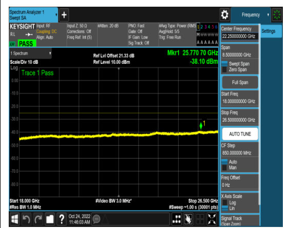
1-N41-PC3-30-90-L-4-N/A-DFT-QPSK-Edge _1RB_Left-1@0-18000-26500-Ant1-25770.7 0--38.10--25-PASS
