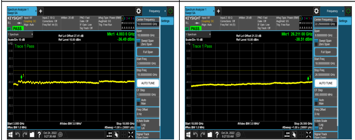
1-N41-PC3-30-20-L-4-N/A-DFT-QPSK-Edge _1RB_Left-1@0-3000-18000-Ant1-4003.00-- 36.49--25-PASS 1-N41-PC3-30-20-L-4-N/A-DFT-QPSK-Edge _1RB_Left-1@0-18000-26500-Ant1-26211.00 --38.51--25-PASS
