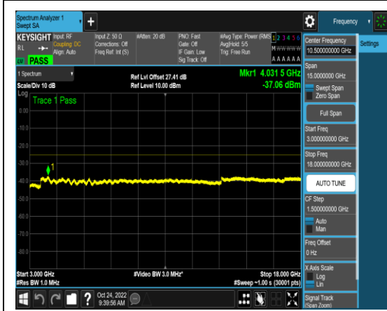
1-N41-PC3-30-30-L-4-N/A-DFT-QPSK-Edge _1RB_Left-1@0-3000-18000-Ant1-4031.50-- 37.06--25-PASS
