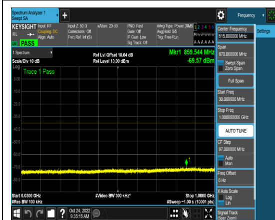
1-N41-PC3-30-20-H-4-N/A-DFT-QPSK-Edge _1RB_Left-1@0-30-1000-Ant1-859.54--69.57 --35-PASS
