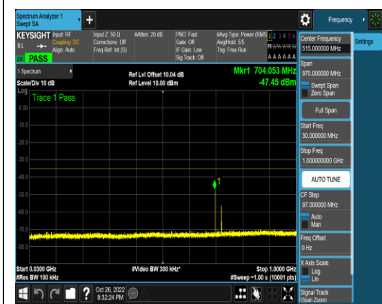
1-N41-PC3-30-15-H-16-N/A-CP-QPSK-Edge _1RB_Left-1@0-30-1000-Ant1-704.05--47.45 --35-PASS
