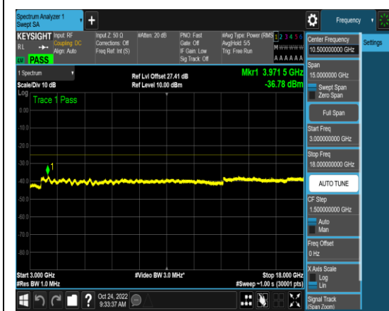
1-N41-PC3-30-20-M-16-N/A-CP-QPSK-Edge _1RB_Left-1@0-3000-18000-Ant1-3971.50-- 36.78--25-PASS
