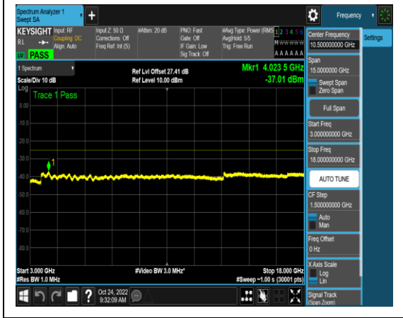
1-N41-PC3-30-20-M-4-N/A-DFT-QPSK-Edge _1RB_Left-1@0-3000-18000-Ant1-4023.50-- 37.01--25-PASS
