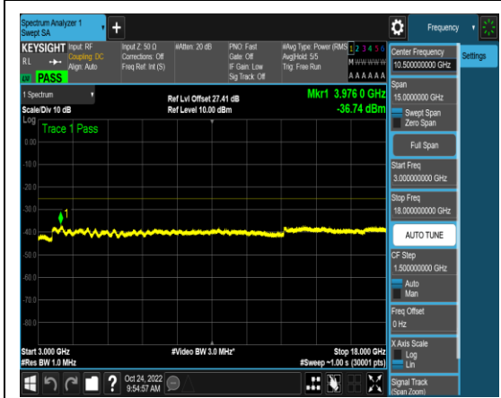
1-N41-PC3-30-40-M-4-N/A-DFT-QPSK-Edge _1RB_Left-1@0-3000-18000-Ant1-3976.00-- 36.74--25-PASS
