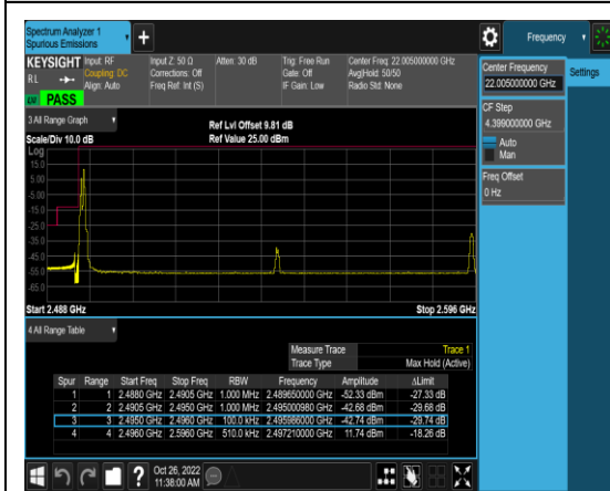
1-N41-PC3-30-100-L-1-DFT-PI2BPSK-Edge_1RB_Left-1 @0-Ant1-1-X:2489.65MHz
