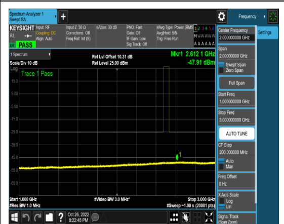
1-N41-PC3-30-15-L-16-N/A-CP-QPSK-Edge _1RB_Left-1@0-1000-3000-Ant1-2612.10--4 7.91--25-PASS
