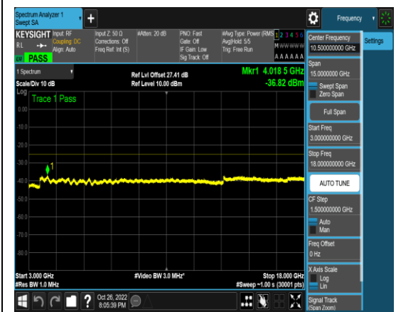
1-N41-PC3-30-10-L-4-N/A-DFT-QPSK-Edge _1RB_Left-1@0-3000-18000-Ant1-4018.50-- 36.82--25-PASS
