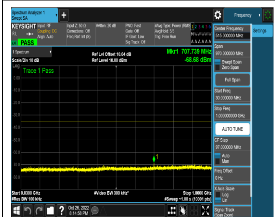
1-N41-PC3-30-10-H-4-N/A-DFT-QPSK-Edge _1RB_Left-1@0-30-1000-Ant1-707.74--68.68 --35-PASS
