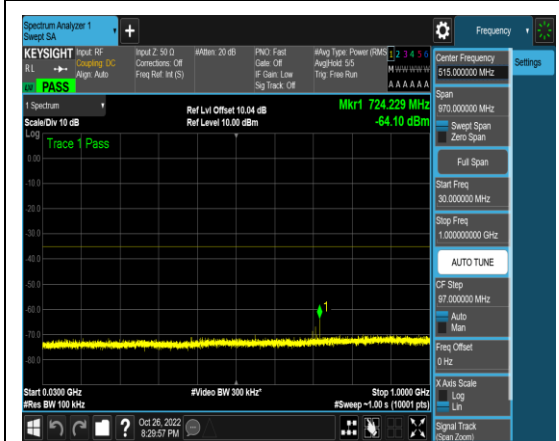
1-N41-PC3-30-15-H-4-N/A-DFT-QPSK-Edge _1RB_Left-1@0-30-1000-Ant1-724.23--64.10 --35-PASS
