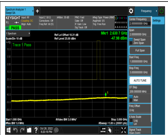
1-N41-PC3-30-15-L-4-N/A-DFT-QPSK-Edge _1RB_Left-1@0-1000-3000-Ant1-2630.70--4 7.98--25-PASS
