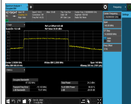
1-N41-PC3-30-70-M-5-CP-QPSK-Outer_Full- 189@0-Ant1-67.332-73.01-≤70-PASS
