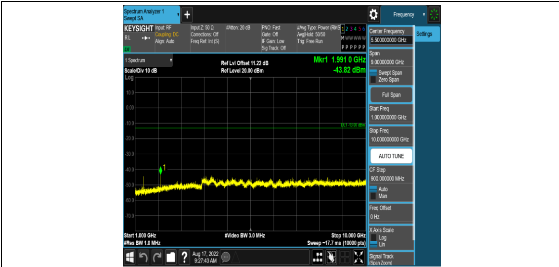
Band71-10MHz-QPSK-133172-1RB#0-Range4: 1000~10000MHz
