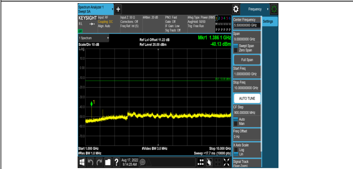
Band71-5MHz-QPSK-133447-1RB#0-Range4:1000~10000MHz
