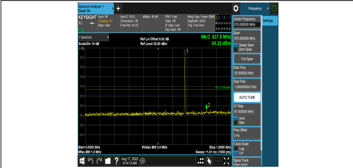
Band71-5MHz-QPSK-133447-1RB#0-Range3:30~1000MHz
