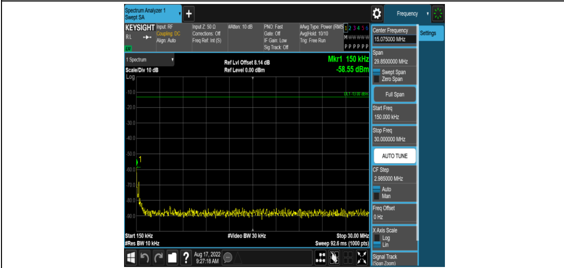
Band71-10MHz-QPSK-133172-1RB#0-Range2:0.15~30MHz
