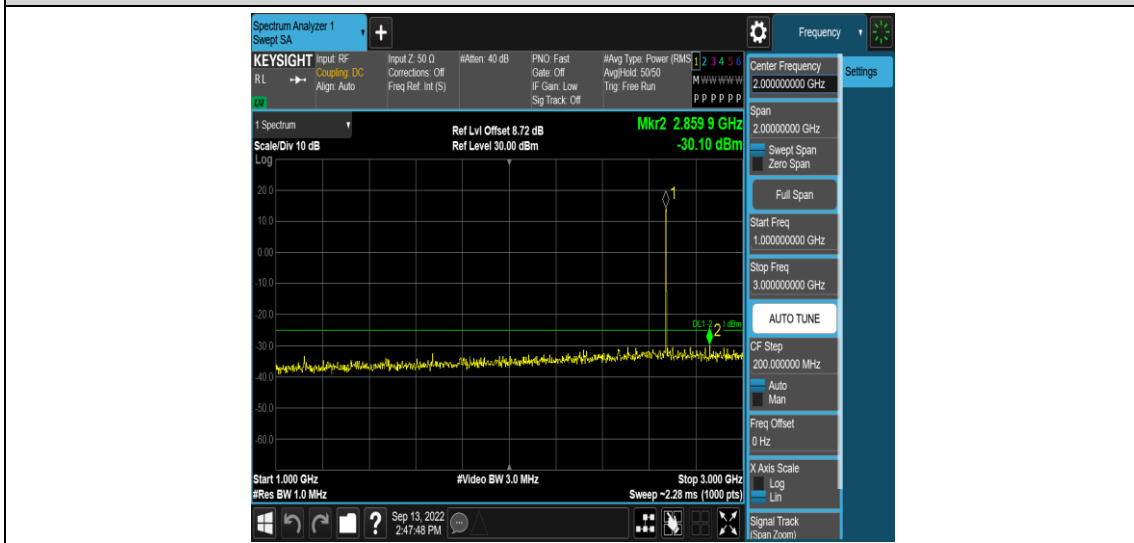
Band41-20MHz-QPSK-41490-1RB#0-Range4:1000~3000MHz
