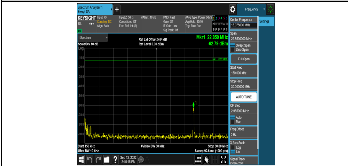
Band41-20MHz-QPSK-40620-1RB#0-Range2:0.15~30MHz
