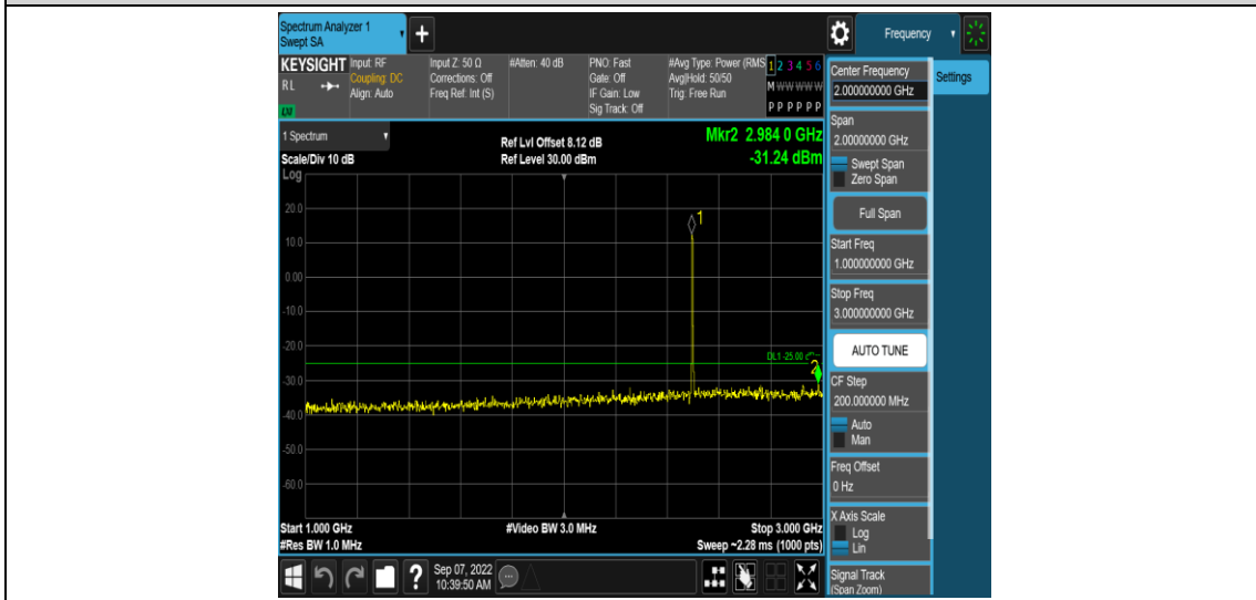
Band41-5MHz-QPSK-39675-1RB#0-Range4:1000~3000MHz
