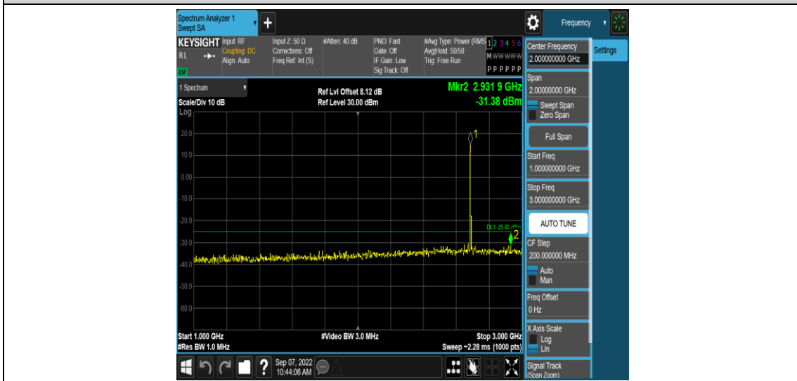
Band41-5MHz-QPSK-41565-1RB#0-Range4:1000~3000MHz
