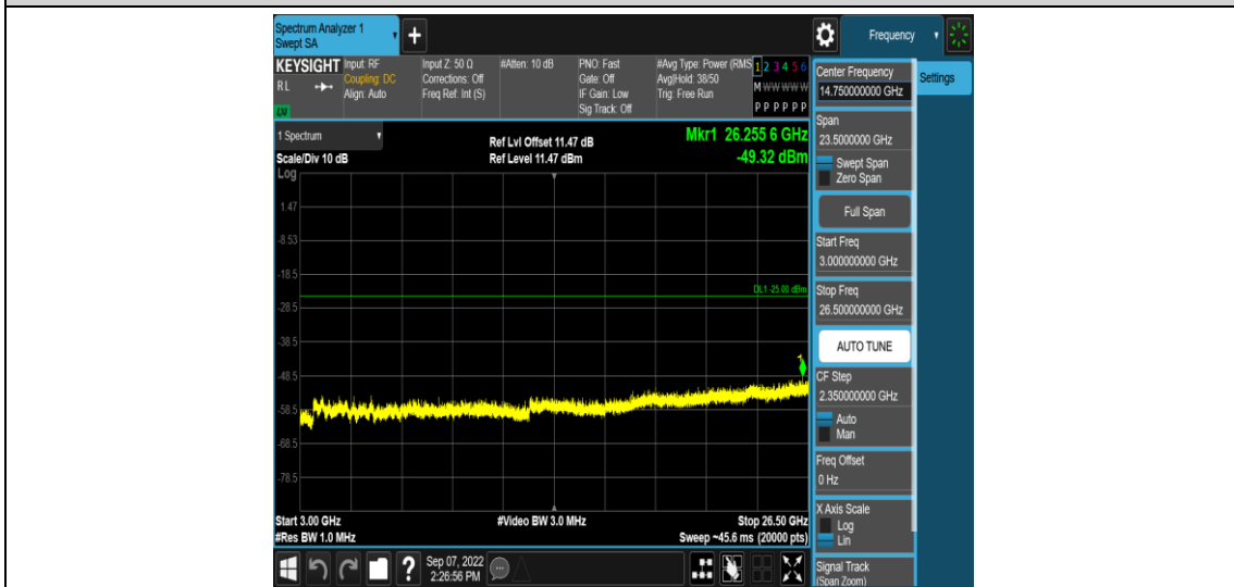
Band41-10MHz-QPSK-39700-1RB#0-Range5:3000~26500MHz
