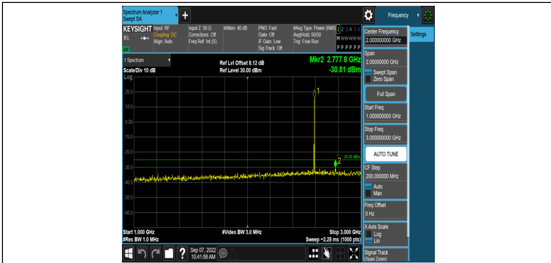
Band41-5MHz-QPSK-40620-1RB#0-Range4:1000~3000MHz
