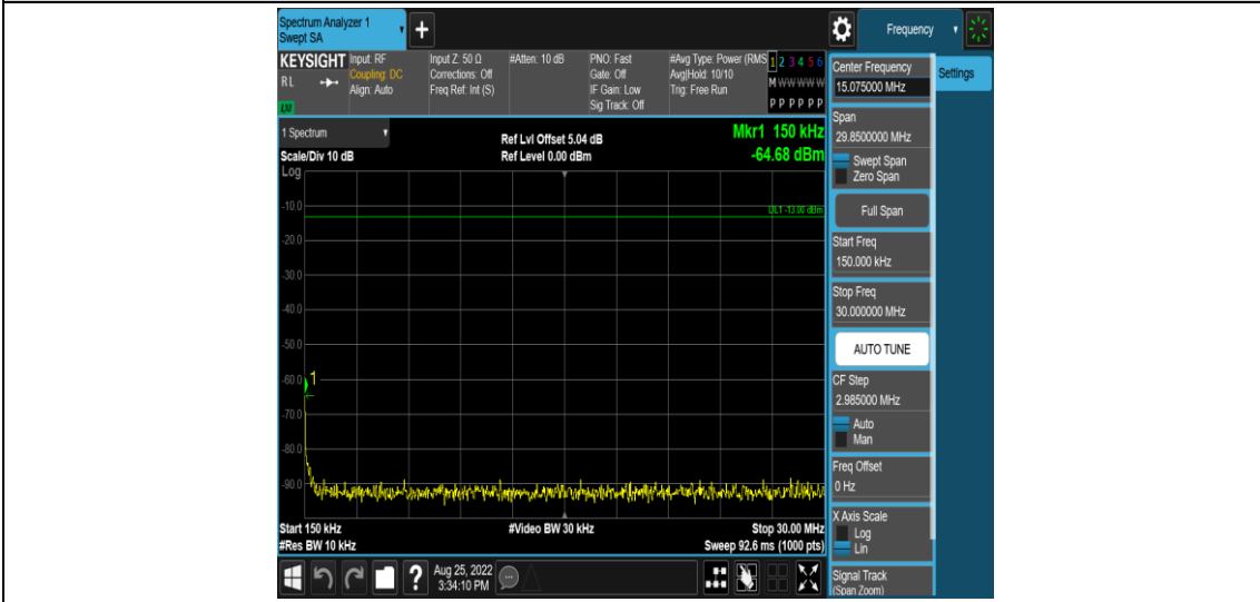
Band26-3MHz-QPSK-27025-1RB#0-Range2:0.15~30MHz
