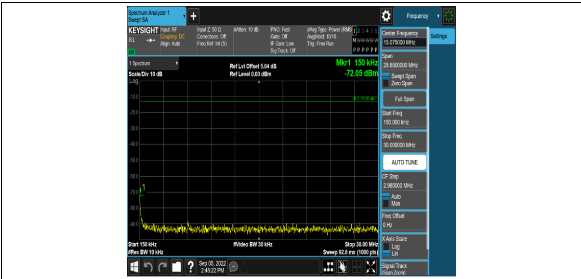
Band25-20MHz-QPSK-26140-1RB#0-Range2:0.15~30MHz
