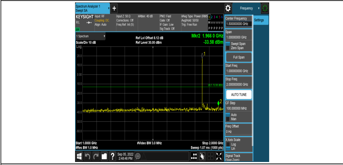
Band25-20MHz-QPSK-26140-1RB#0-Range4:1000~2000MHz
