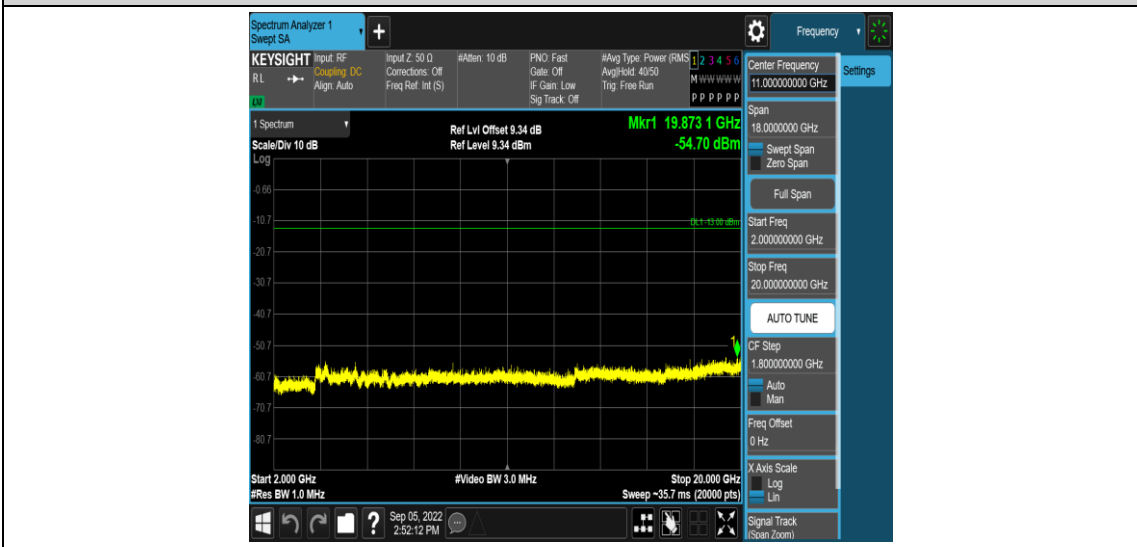
Band25-20MHz-16QAM-26365-1RB#0-Range5:2000~20000MHz
