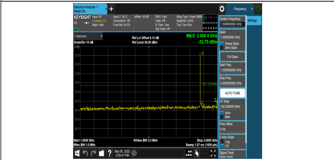
Band25-15MHz-QPSK-26365-1RB#0-Range4:1000~2000MHz
