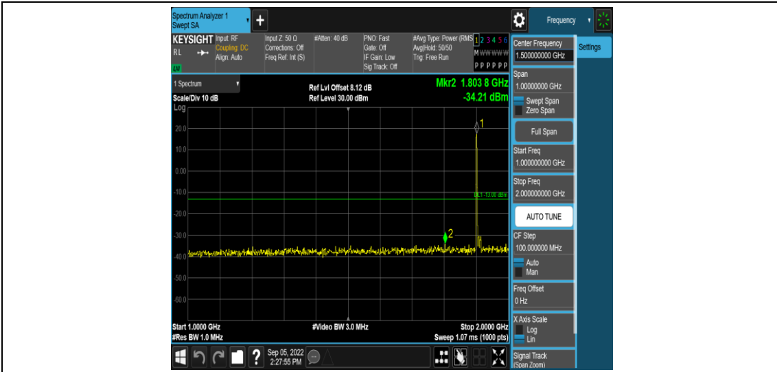
Band25-15MHz-QPSK-26615-1RB#0-Range4:1000~2000MHz
