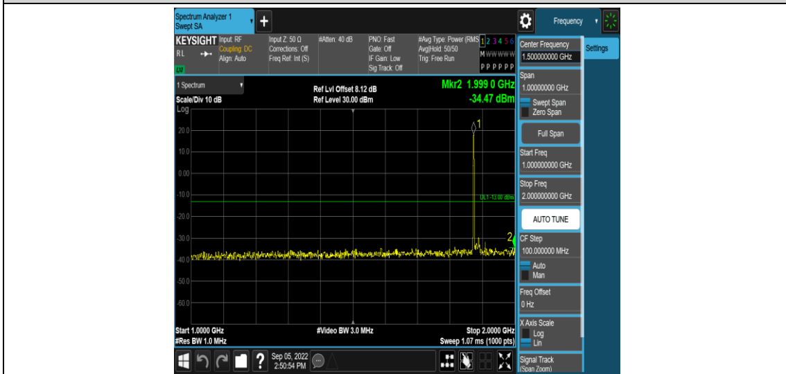
Band25-20MHz-QPSK-26365-1RB#0-Range4:1000~2000MHz
