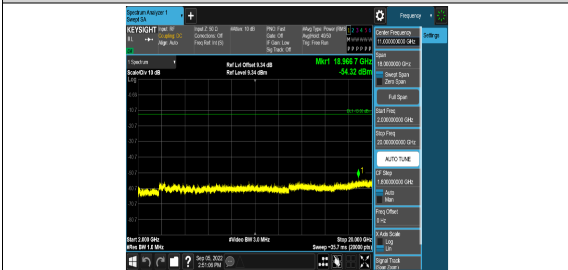
Band25-20MHz-QPSK-26365-1RB#0-Range5:2000~20000MHz
