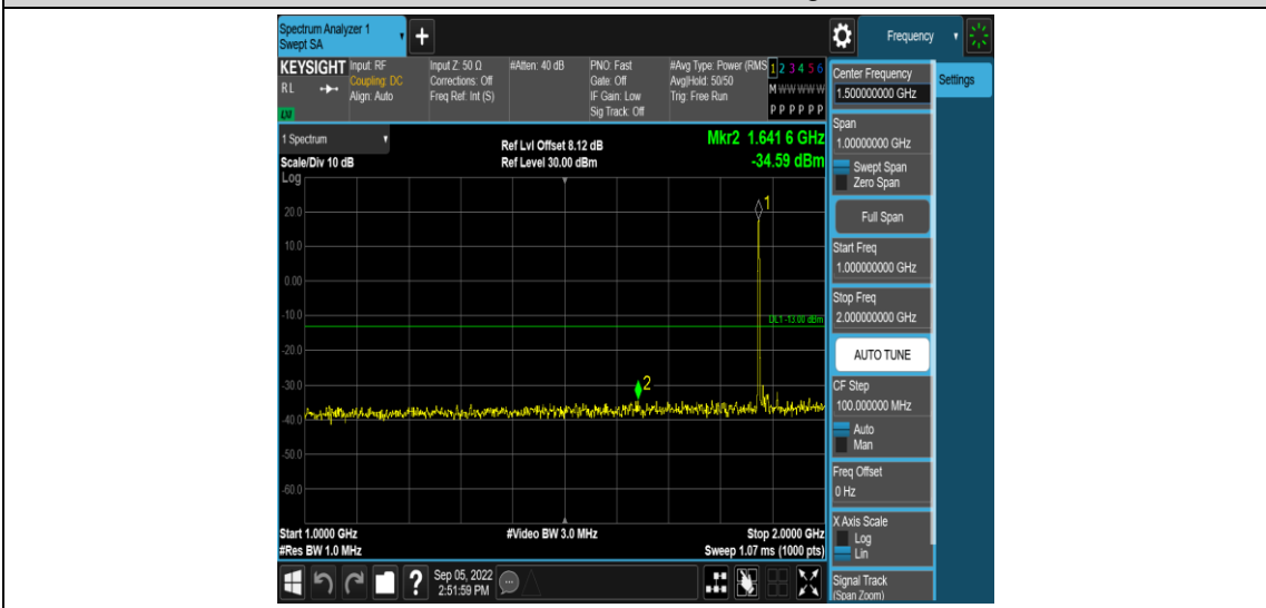
Band25-20MHz-16QAM-26365-1RB#0-Range4:1000~2000MHz
