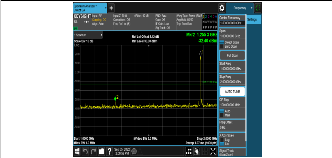
Band25-10MHz-QPSK-26365-1RB#0-Range4:1000~2000MHz
