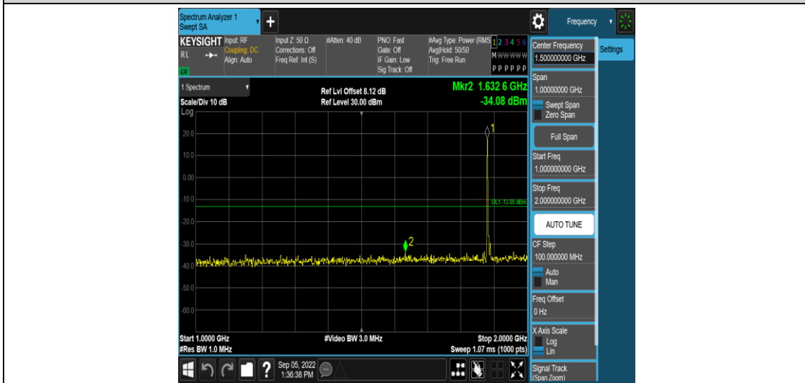
Band25-5MHz-QPSK-26365-1RB#0-Range4:1000~2000MHz
