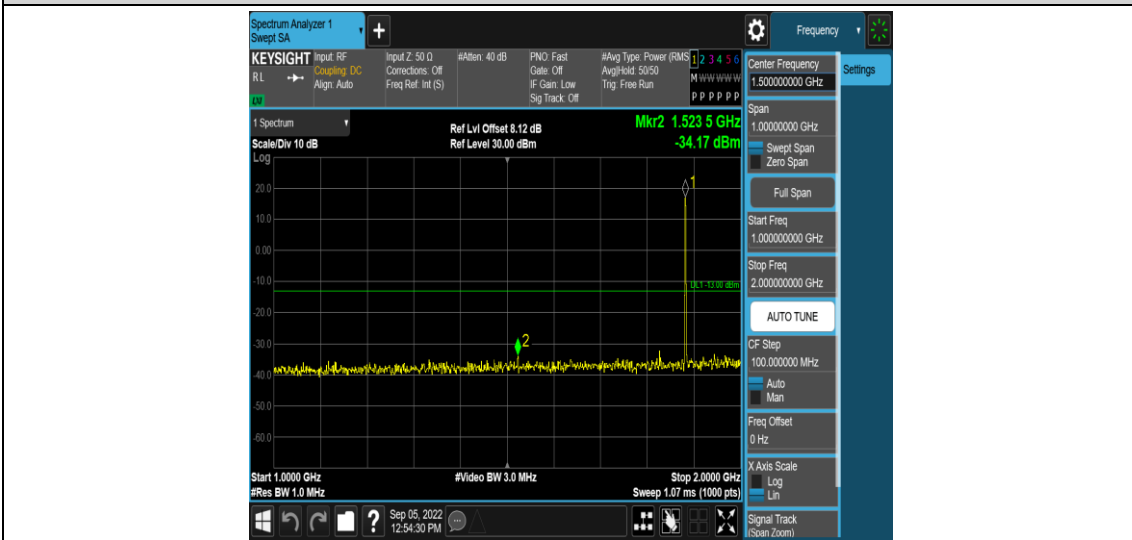
Band25-1.4MHz-QPSK-26365-1RB#0-Range4:1000~2000MHz
