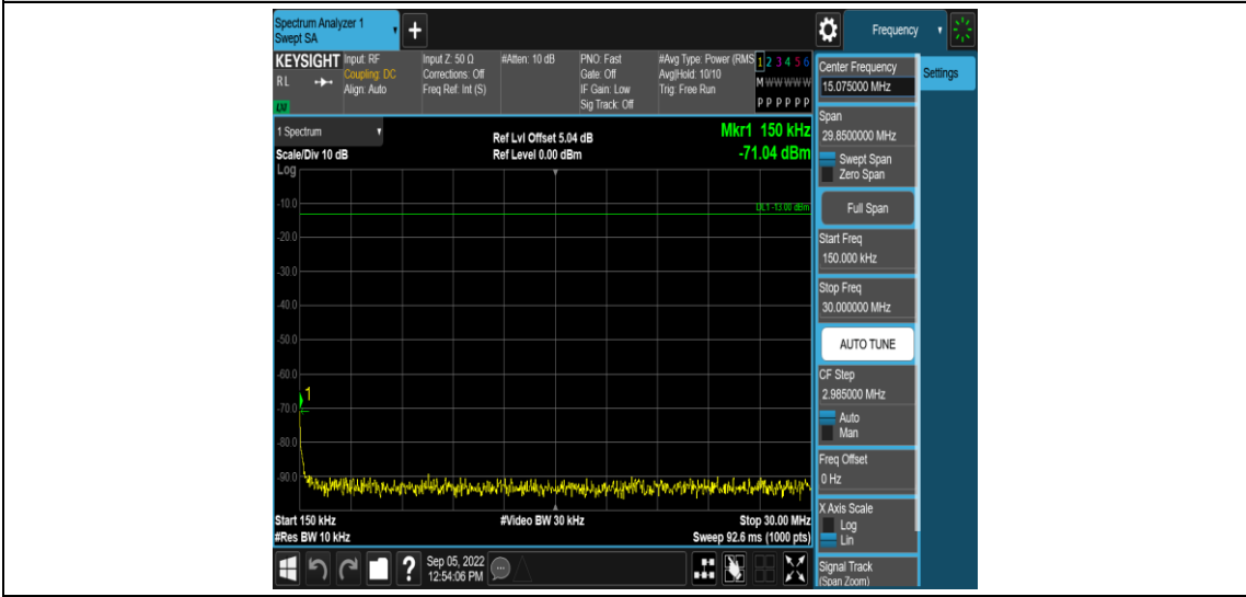
Band25-1.4MHz-QPSK-26365-1RB#0-Range2:0.15~30MHz
