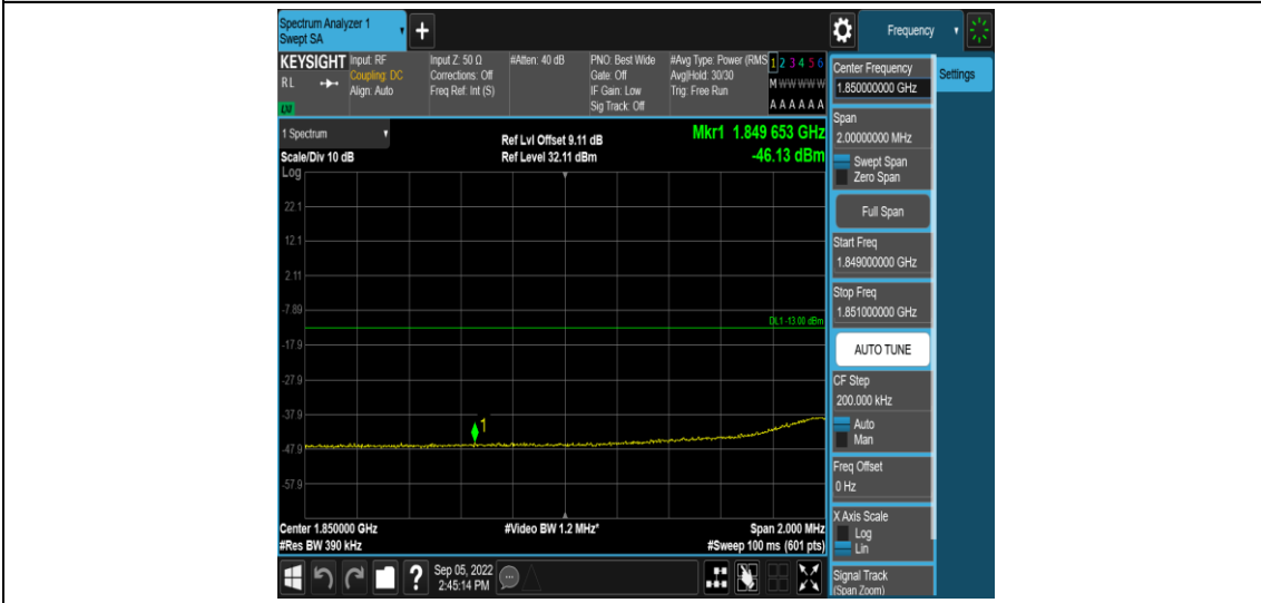
Band25-20MHz-QPSK-26140-1RB#99
