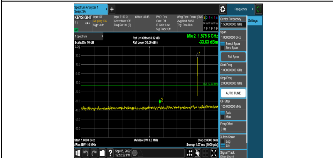
Band25-1.4MHz-QPSK-26047-1RB#0-Range4:1000~2000MHz
