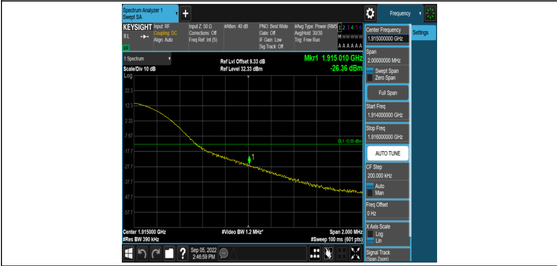
Band25-20MHz-QPSK-26590-1RB#90
