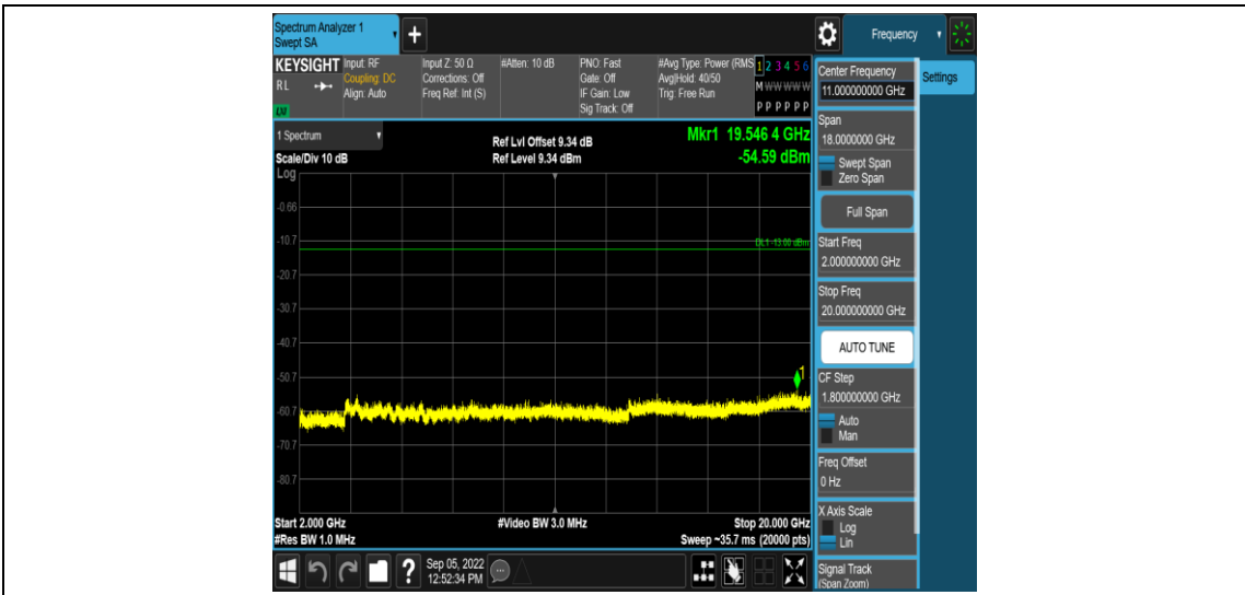
Band25-1.4MHz-QPSK-26047-1RB#0-Range5:2000~20000MHz
