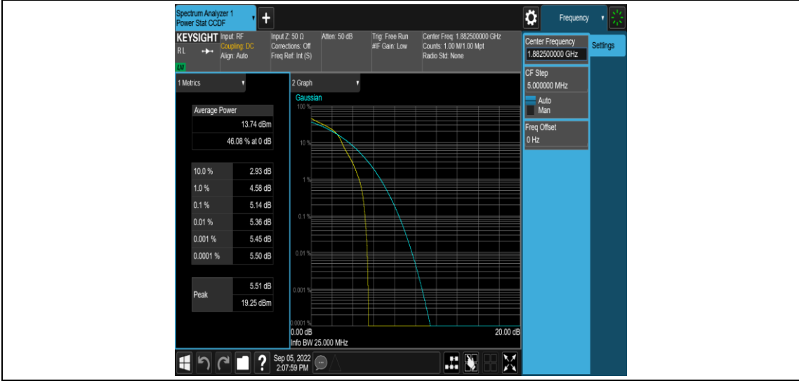
Band25-10MHz-16QAM-26365-1RB#0
