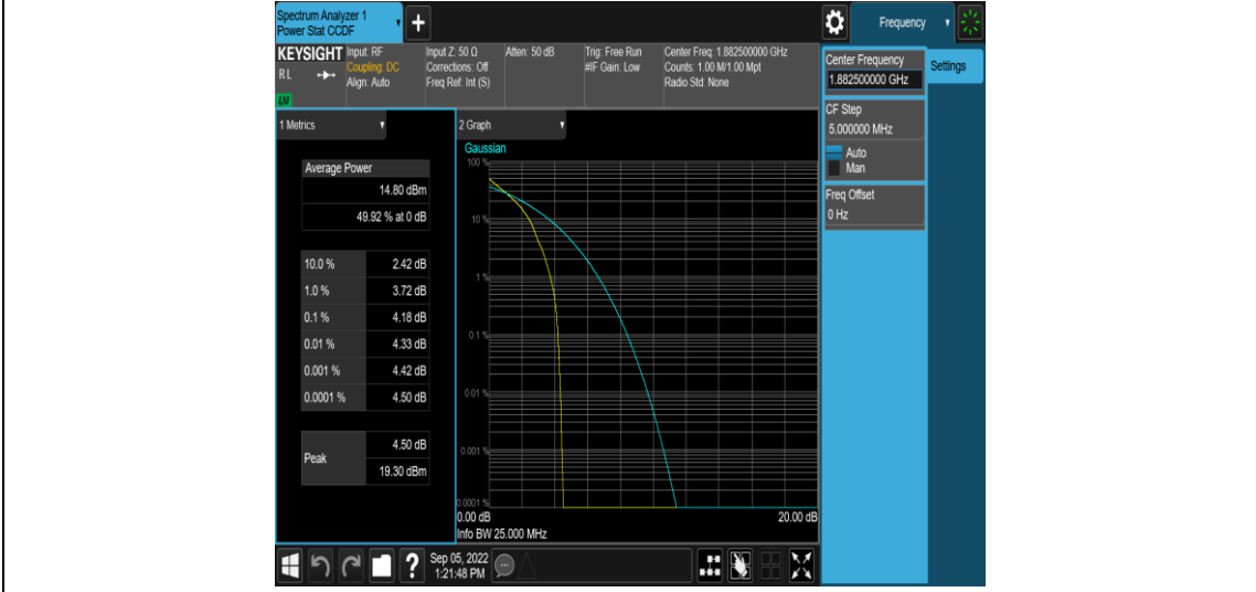
Band25-3MHz-QPSK-26365-1RB#0
