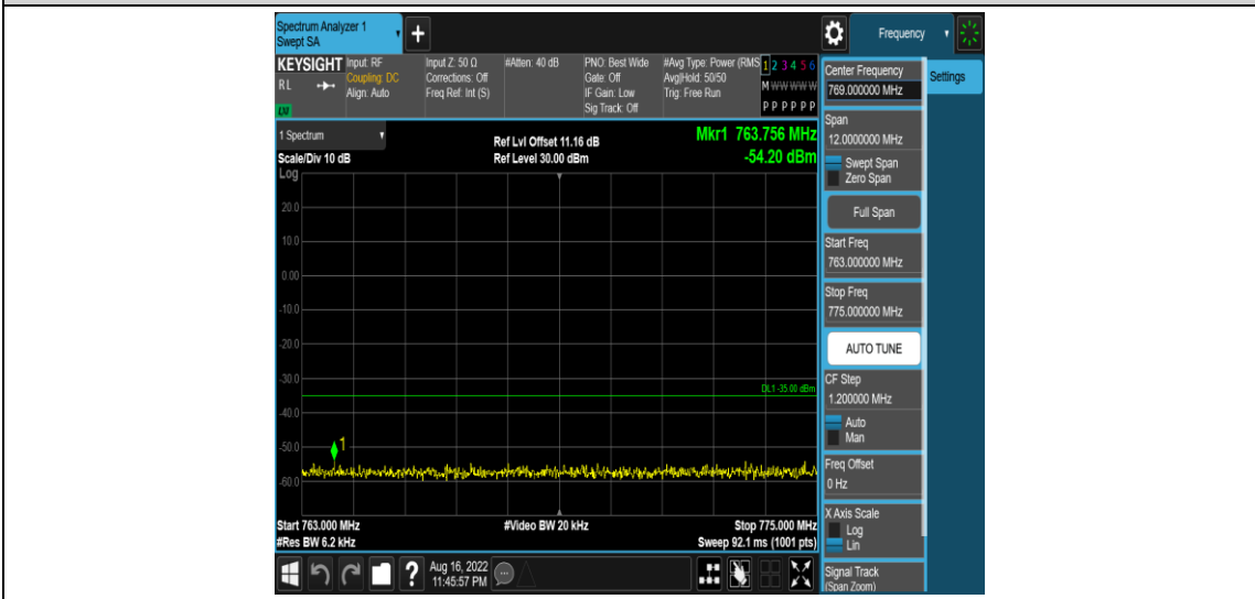
Band13-5MHz-QPSK-23255-1RB#0-Range5:763~775MHz
