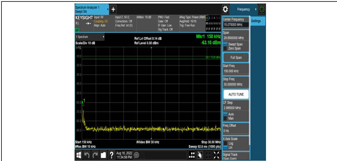
Band13-5MHz-QPSK-23205-1RB#0-Range2:0.15~30MHz
