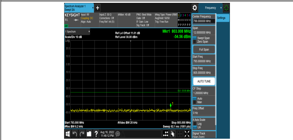
Band13-5MHz-QPSK-23255-1RB#0-Range6:793~805MHz
