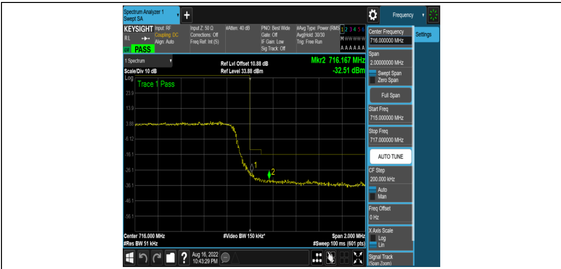
Band12-3MHz-QPSK-23165-15RB#0
