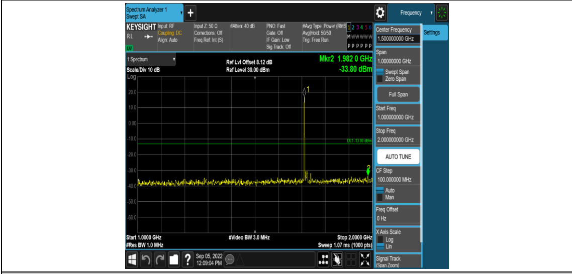
Band4-15MHz-QPSK-2025-1RB#0-Range4:1000~2000MHz
