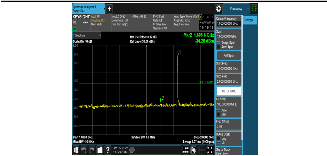
Band4-3MHz-QPSK-20175-1RB#0-Range4:1000~2000MHz
