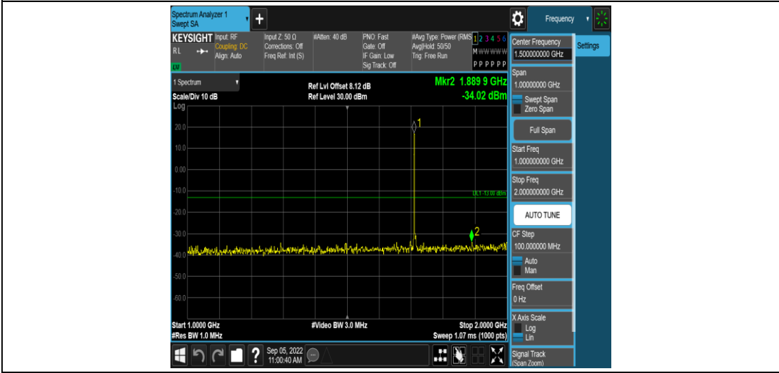
Band4-3MHz-QPSK-19965-1RB#0-Range4:1000~2000MHz
