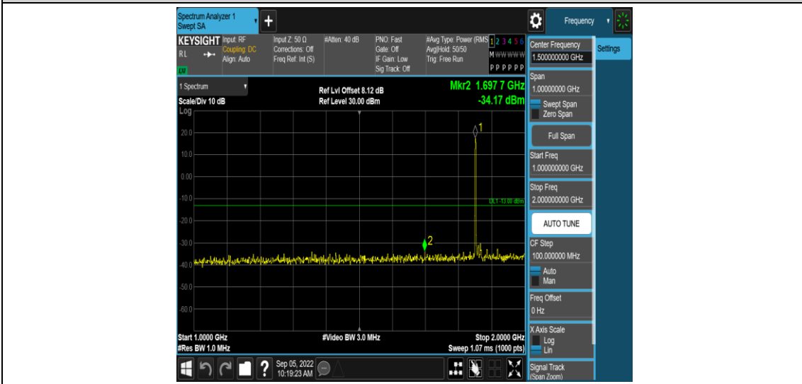
Band2-20MHz-QPSK-18700-1RB#0-Range4:1000~2000MHz
