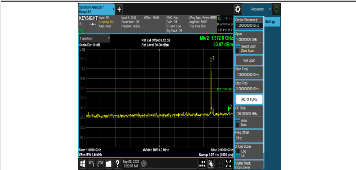
Band2-10MHz-QPSK-18650-1RB#0-Range4:1000~2000MHz
