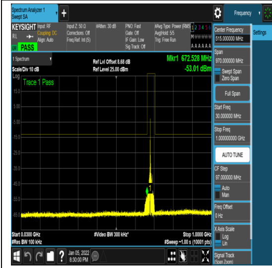
1-N71-PC3-15-10-H-16-CP-QPSK-Edge_1R B_Left-1@0-0.000-0.000--53.01--33-PASS
