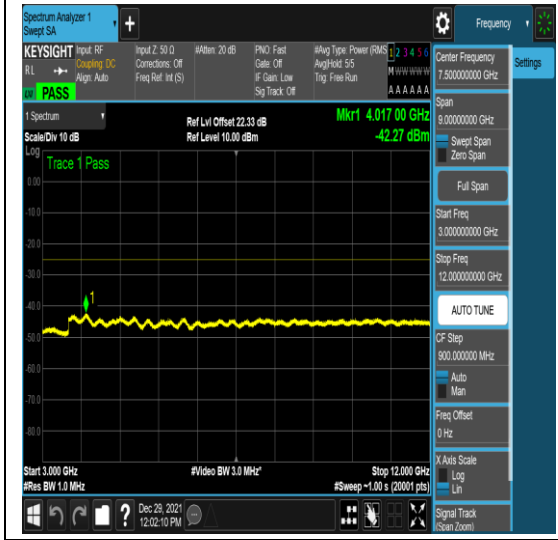
n41-PC3-30-60-L-4-N/A-N/A-N/A-DFT-QPSK -Edge_1RB_Left-1@0-3000-12000--42.27--2 5-PASS
