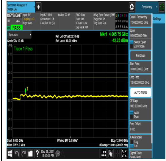
n41-PC3-30-100-M-4-N/A-N/A-N/A-DFT-QPS K-Edge_1RB_Left-1@0-3000-12000--42.25-- 25-PASS
