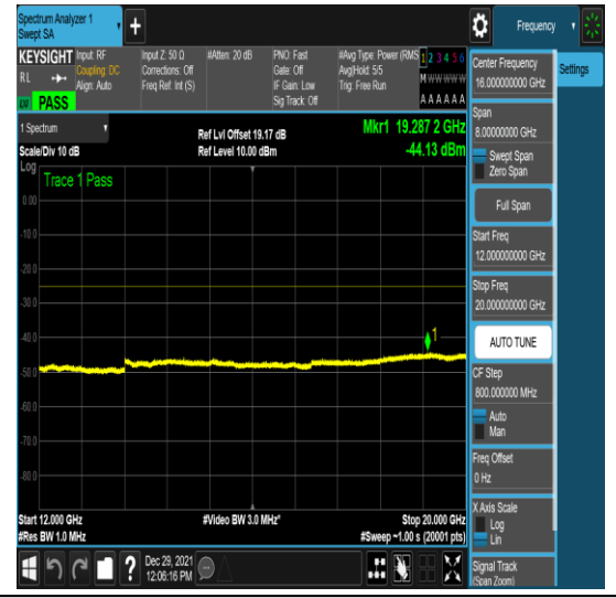
n41-PC3-30-60-M-4-N/A-N/A-N/A-DFT-QPS K-Edge_1RB_Left-1@0-12000-20000--44.13 --25-PASS
