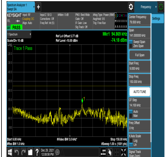
n41-PC3-30-60-H-4-N/A-N/A-N/A-DFT-QPSK -Edge_1RB_Left-1@0-0.009-0.15--74.18--55 -PASS
