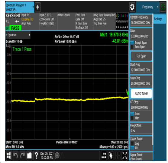
n41-PC3-30-60-L-4-N/A-N/A-N/A-DFT-QPSK -Edge_1RB_Left-1@0-12000-20000--43.81-- 25-PASS
