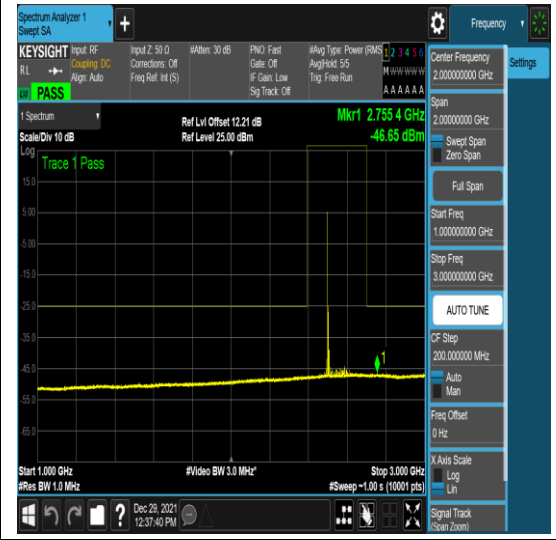
n41-PC3-30-100-L-16-N/A-N/A-N/A-CP-QPS K-Edge_1RB_Left-1@0-1000-3000--46.65--2 5-PASS
