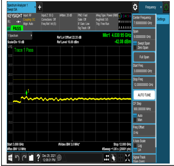
n41-PC3-30-60-M-4-N/A-N/A-N/A-DFT-QPS K-Edge_1RB_Left-1@0-3000-12000--42.08-- 25-PASS
