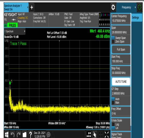
n41-PC3-30-90-M-4-N/A-N/A-N/A-DFT-QPSK K-Edge_1RB_Left-1@0-0.15-30--66.08--45-PASS
