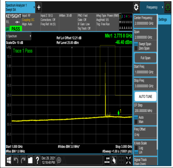
n41-PC3-30-80-M-16-N/A-N/A-N/A-CP-QPS K-Edge_1RB_Left-1@0-1000-3000--46.40--2 5-PASS
