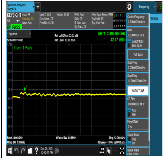
n41-PC3-30-90-H-4-N/A-N/A-N/A-DFT-QPSK -Edge_1RB_Left-1@0-3000-12000--42.47--2 5-PASS
