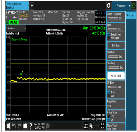
n41-PC3-30-80-M-4-N/A-N/A-N/A-DFT-QPS K-Edge_1RB_Left-1@0-3000-12000--42.19-- 25-PASS
