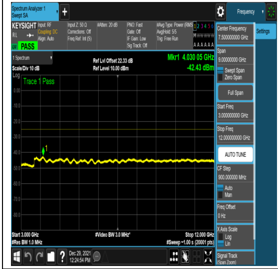
n41-PC3-30-90-L-4-N/A-N/A-N/A-DFT-QPSK -Edge_1RB_Left-1@0-3000-12000--42.43--2 5-PASS
