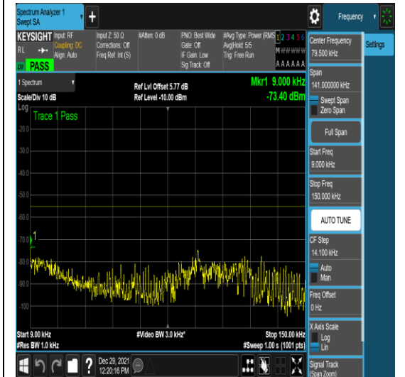
n41-PC3-30-80-H-4-N/A-N/A-N/A-DFT-QPSK -Edge_1RB_Left-1@0-0.009-0.15--73.40--55 -PASS
