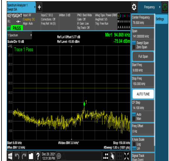
n41-PC3-30-90-H-4-N/A-N/A-N/A-DFT-QPSK -Edge_1RB_Left-1 @0-0.009-0.15--75.04--55 -PASS
