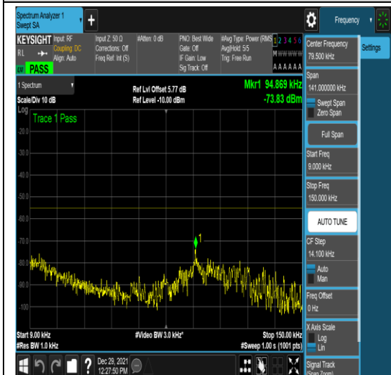
n41-PC3-30-90-M-4-N/A-N/A-N/A-DFT-QPSK K-Edge_1RB_Left-1@0-0.009-0.15--73.83--55-PASS
