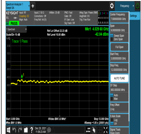
n41-PC3-30-50-H-4-N/A-N/A-N/A-DFT-QPSK -Edge_1RB_Left-1@0-3000-12000--42.04--2 5-PASS
