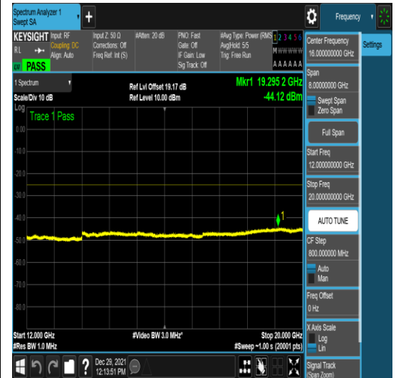
n41-PC3-30-80-L-4-N/A-N/A-N/A-DFT-QPSK -Edge_1RB_Left-1@0-12000-20000--44.12-- 25-PASS
