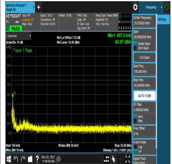
n41-PC3-30-40-H-4-N/A-N/A-N/A-DFT-QPSK -Edge_1RB_Left-1@0-0.15-30--63.97--45-PA SS
