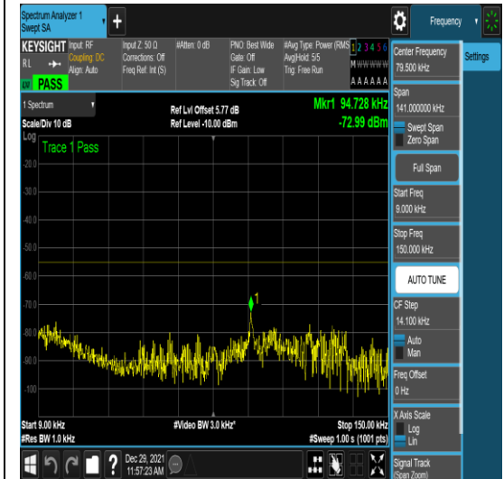
n41-PC3-30-50-H-4-N/A-N/A-N/A-DFT-QPSK -Edge_1RB_Left-1@0-0.009-0.15--72.99--55 -PASS
