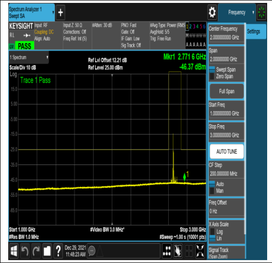
n41-PC3-30-40-H-16-N/A-N/A-N/A-CP-QPSK -Edge_1RB_Left-1@0-1000-3000--46.37--25 -PASS
