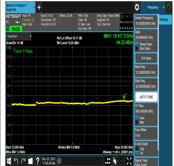
n41-PC3-30-50-H-4-N/A-N/A-N/A-DFT-QPSK -Edge_1RB_Left-1@0-12000-20000--44.23-- 25-PASS
