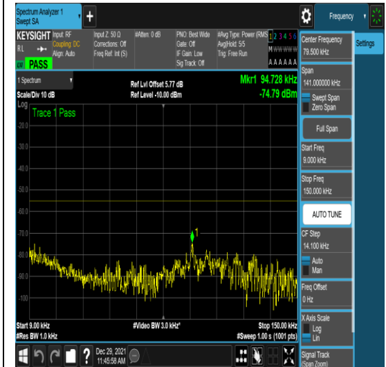
n41-PC3-30-40-H-4-N/A-N/A-N/A-DFT-QPSK -Edge_1RB_Left-1@0-0.009-0.15--74.79--55 -PASS
