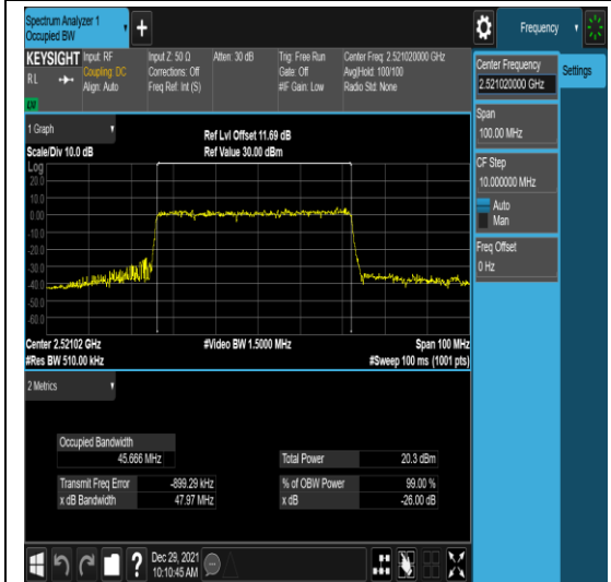
n41-PC3-30-50-L-3-N/A-N/A-N/A-DFT-16QA M-Outer_Full-128@0-Ant1-45.666-47.97-≤50 -PASS
