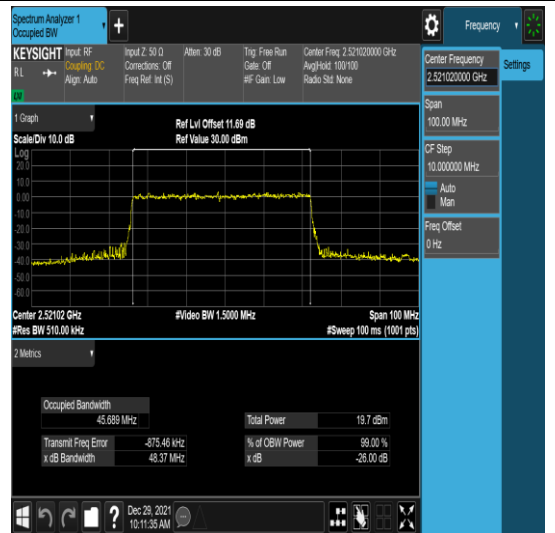
n41-PC3-30-50-L-4-N/A-N/A-N/A-DFT-64QA M-Outer_Full-128@0-Ant1-45.689-48.37-≤50 -PASS
