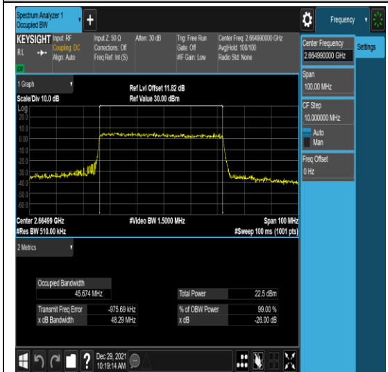
n41-PC3-30-50-H-3-N/A-N/A-N/A-DFT-16QA M-Outer_Full-128@0-Ant1-45.674-48.29-≤50 -PASS
