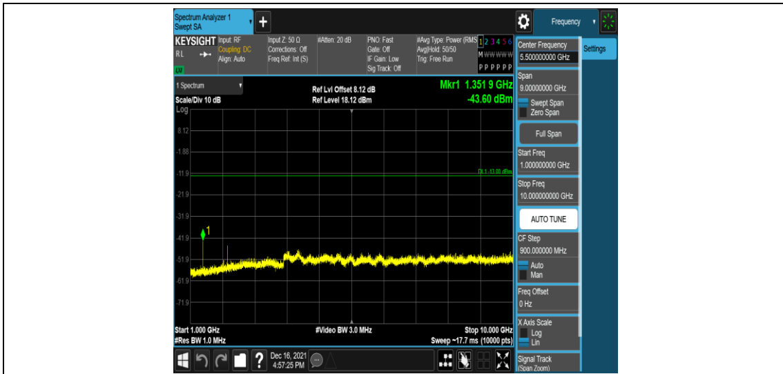
Band71-10MHz-QPSK-133297-1RB#0-Range4:1000~10000MHz
