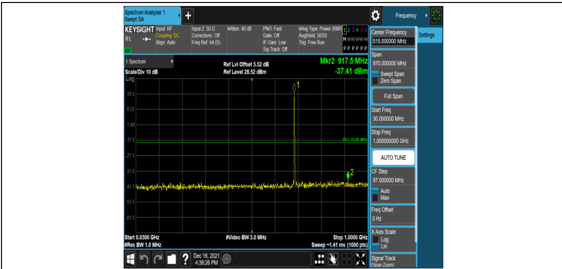
Band71-5MHz-QPSK-133447-1RB#0-Range3:30~1000MHz
