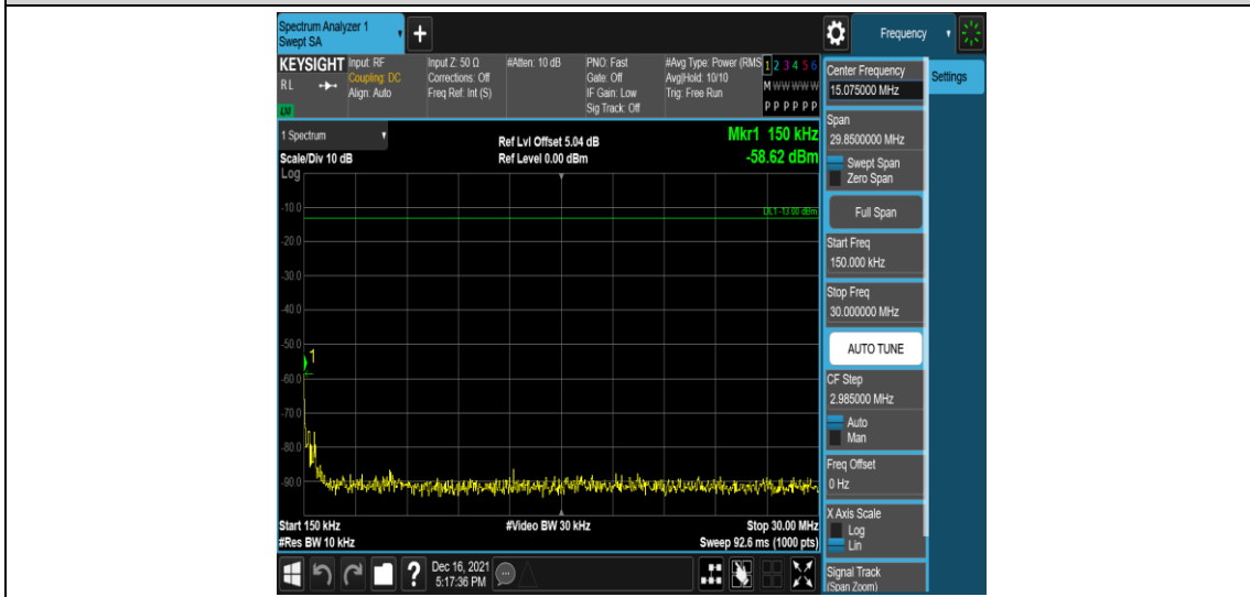
Band71-15MHz-QPSK-133297-1RB#0-Range2:0.15~30MHz
