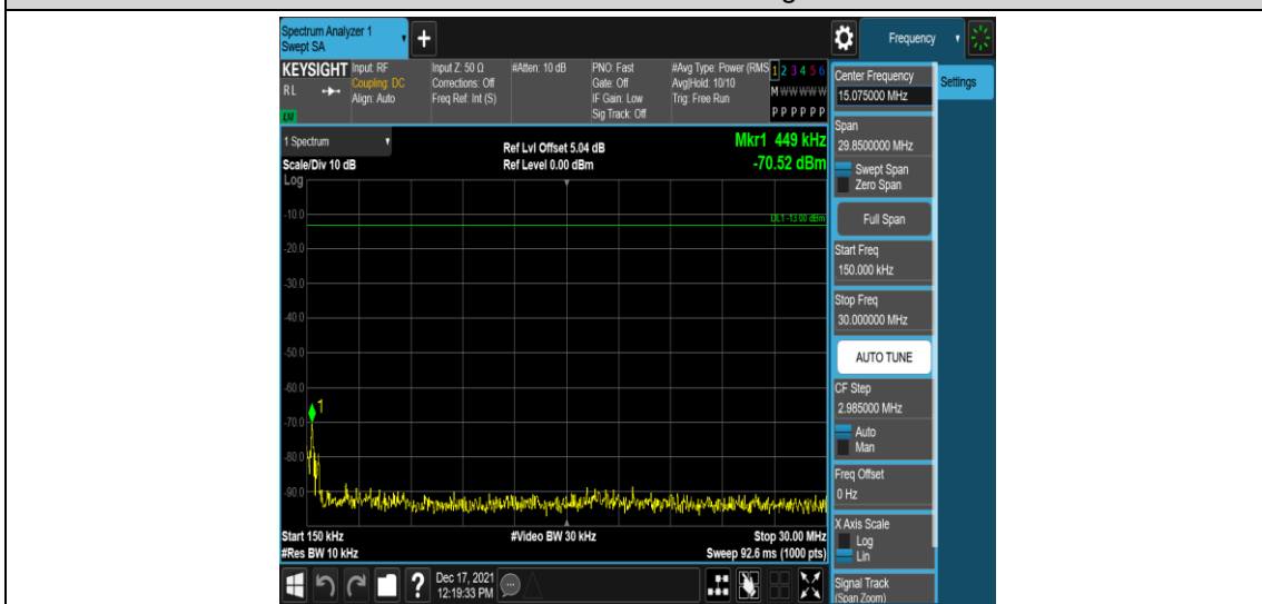
Band41-20MHz-QPSK-39750-1RB#0-Range2:0.15~30MHz
