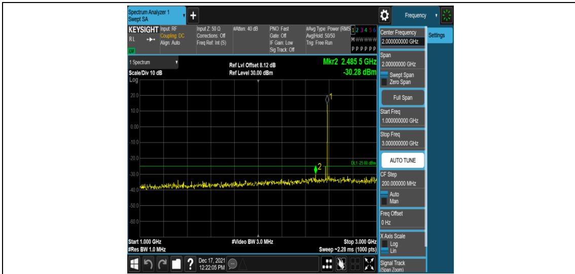
Band41-20MHz-QPSK-40620-1RB#0-Range4:1000~3000MHz
