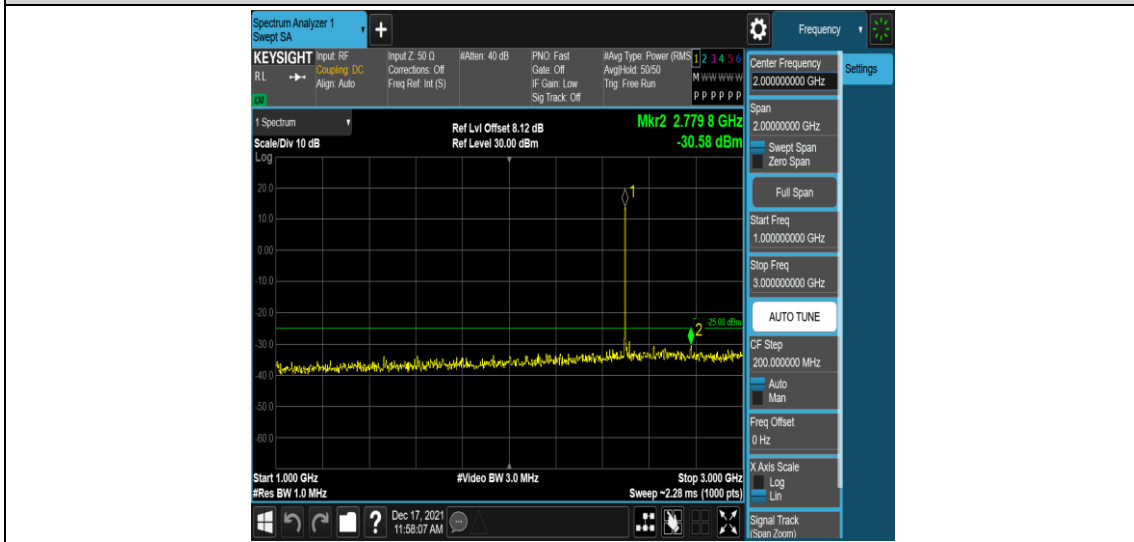
Band41-15MHz-QPSK-39725-1RB#0-Range4:1000~3000MHz
