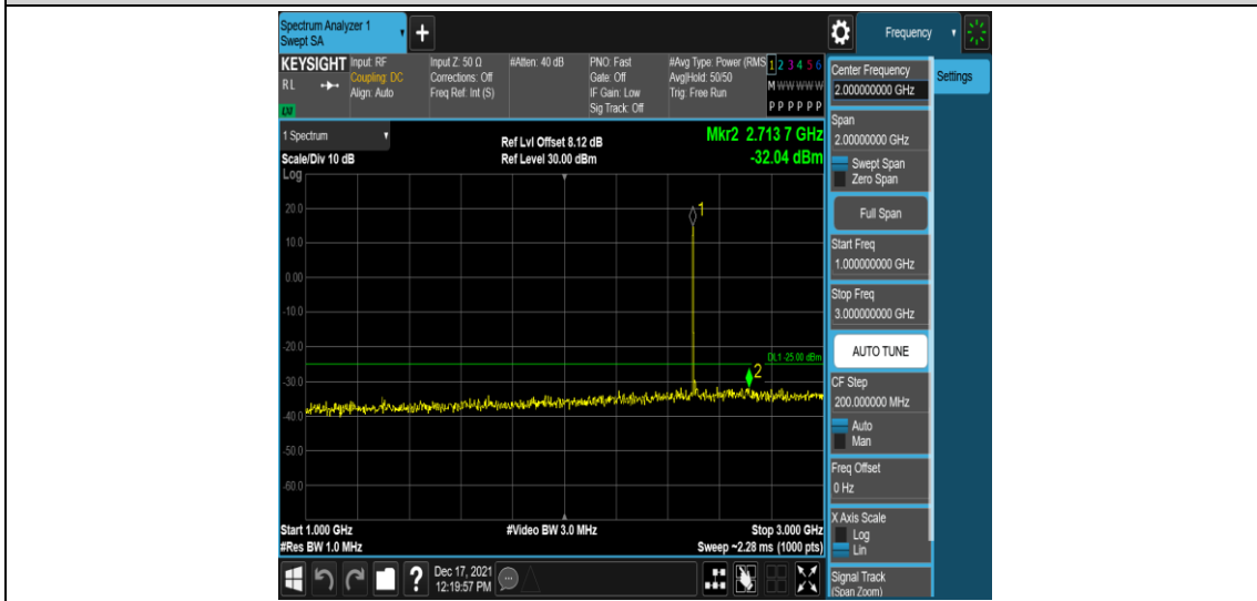
Band41-20MHz-QPSK-39750-1RB#0-Range4:1000~3000MHz
