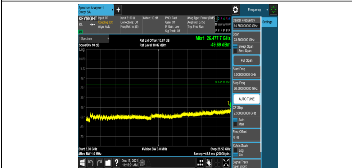
Band41-5MHz-QPSK-39675-1RB#0-Range5:3000~26500MHz
