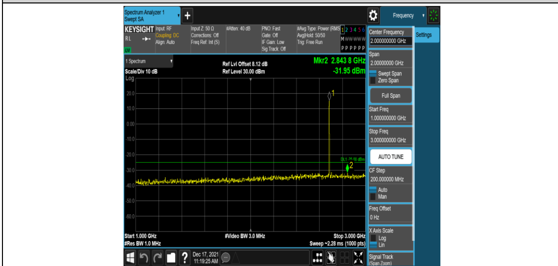
Band41-5MHz-QPSK-41565-1RB#0-Range4:1000~3000MHz
