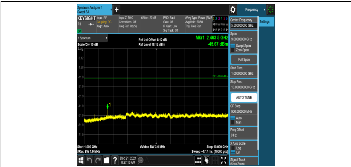
Band26-3MHz-QPSK-26775-1RB#0-Range4:1000~10000MHz
