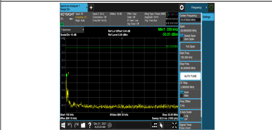
Band26-3MHz-QPSK-26705-1RB#0-Range2:0.15~30MHz
