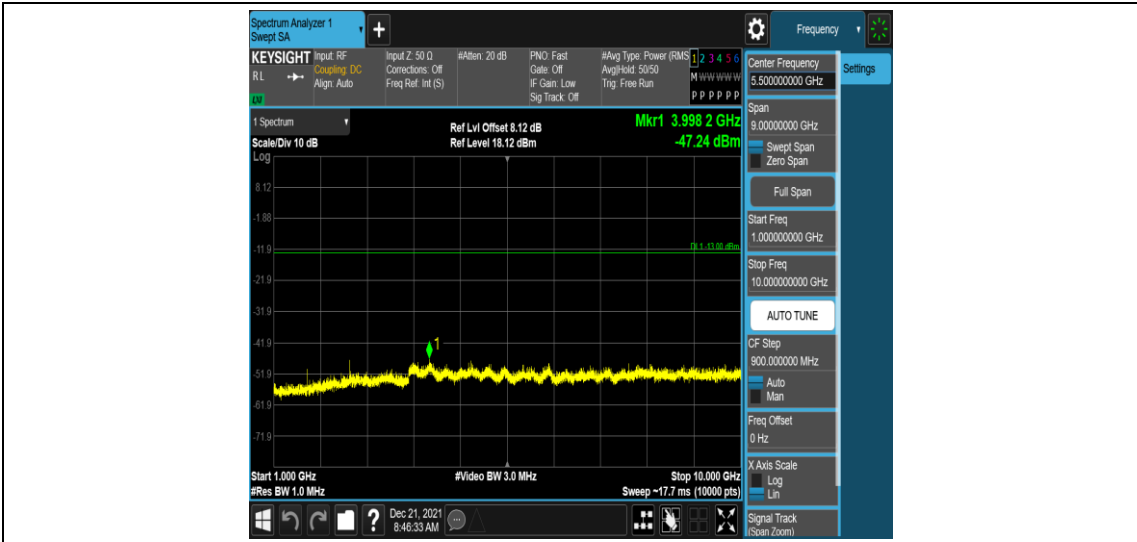
Band26-5MHz-QPSK-26765-1RB#0-Range4:1000~10000MHz
