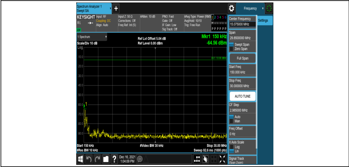
Band25-20MHz-QPSK-26365-1RB#0-Range2:0.15~30MHz
