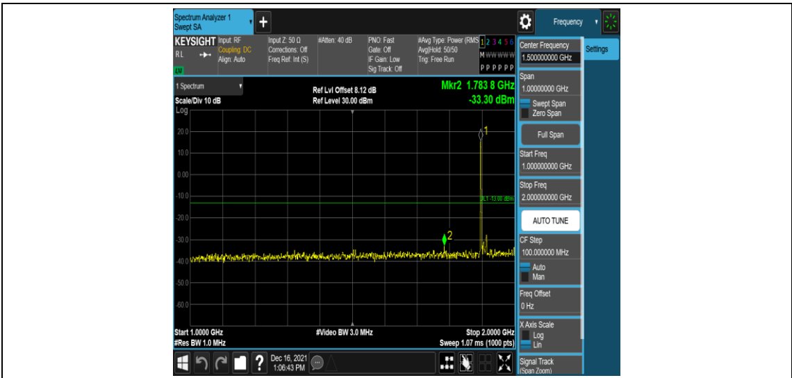
Band25-20MHz-QPSK-26590-1RB#0-Range4:1000~2000MHz
