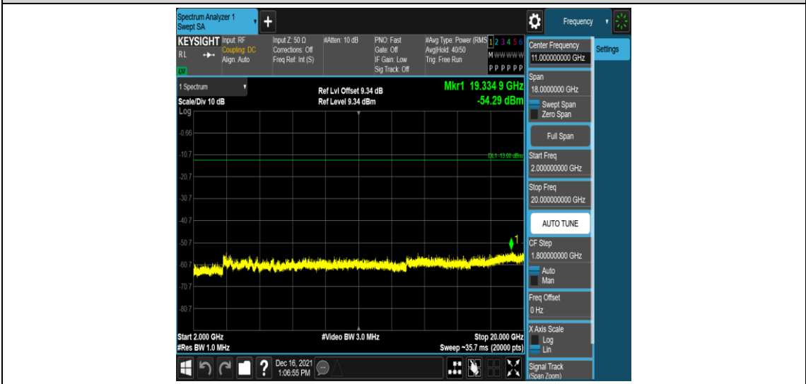
Band25-20MHz-QPSK-26590-1RB#0-Range5:2000~20000MHz
