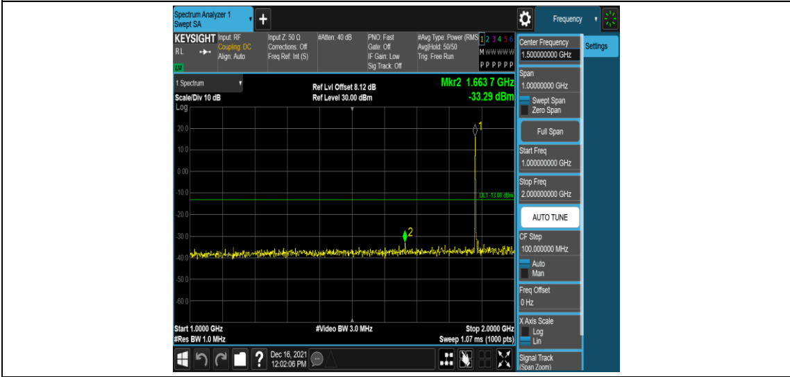
Band25-5MHz-QPSK-26365-1RB#0-Range4:1000~2000MHz
