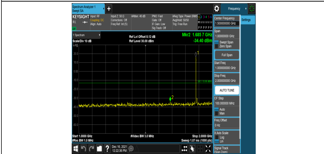
Band25-10MHz-QPSK-26365-1RB#0-Range4:1000~2000MHz
