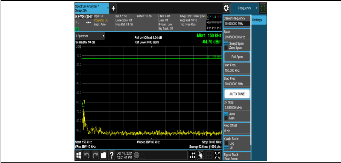
Band25-5MHz-QPSK-26365-1RB#0-Range2:0.15~30MHz
