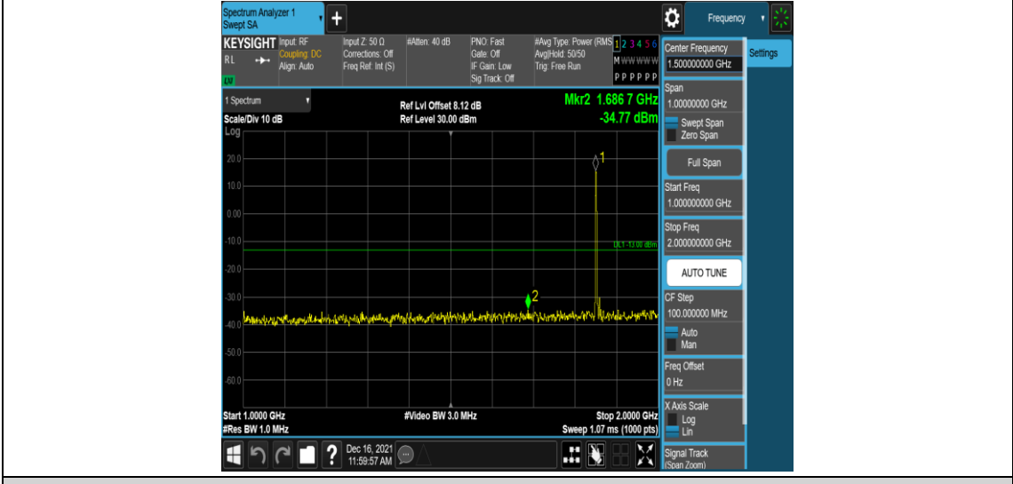
Band25-5MHz-QPSK-26065-1RB#0-Range4:1000~2000MHz
