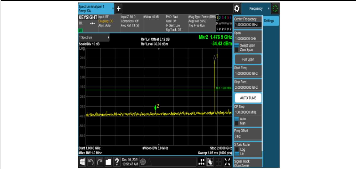
Band25-1.4MHz-QPSK-26365-1RB#0-Range4:1000~2000MHz
