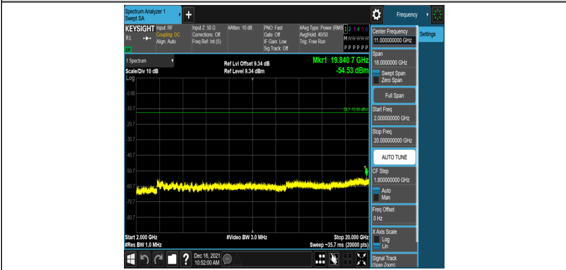
Band25-1.4MHz-QPSK-26365-1RB#0-Range5:2000~20000MHz
