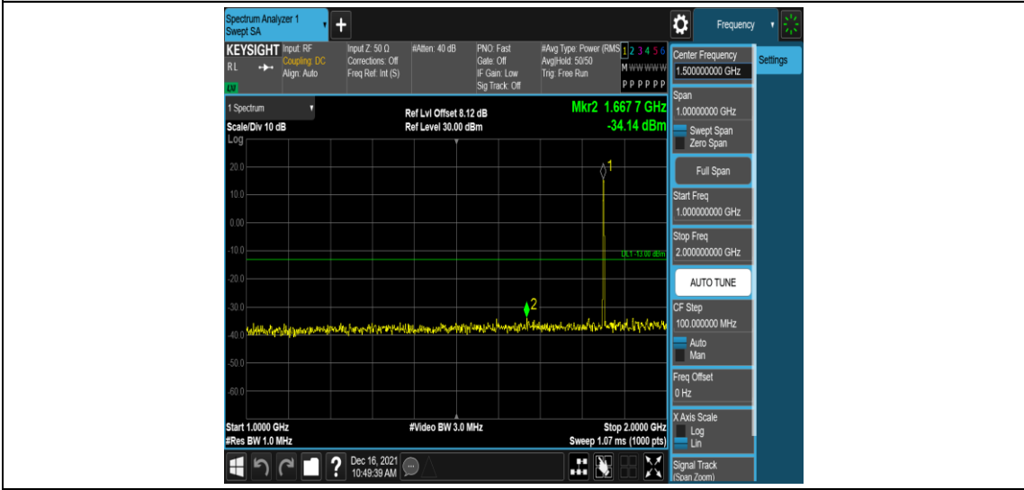
Band25-1.4MHz-QPSK-26047-1RB#0-Range4:1000~2000MHz
