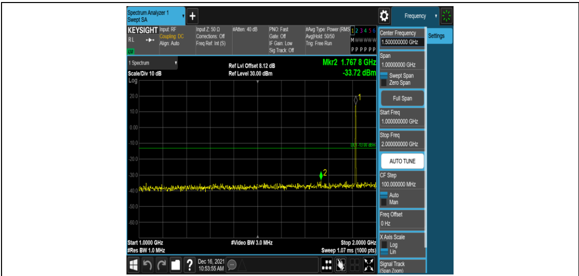
Band25-1.4MHz-QPSK-26683-1RB#0-Range4:1000~2000MHz
