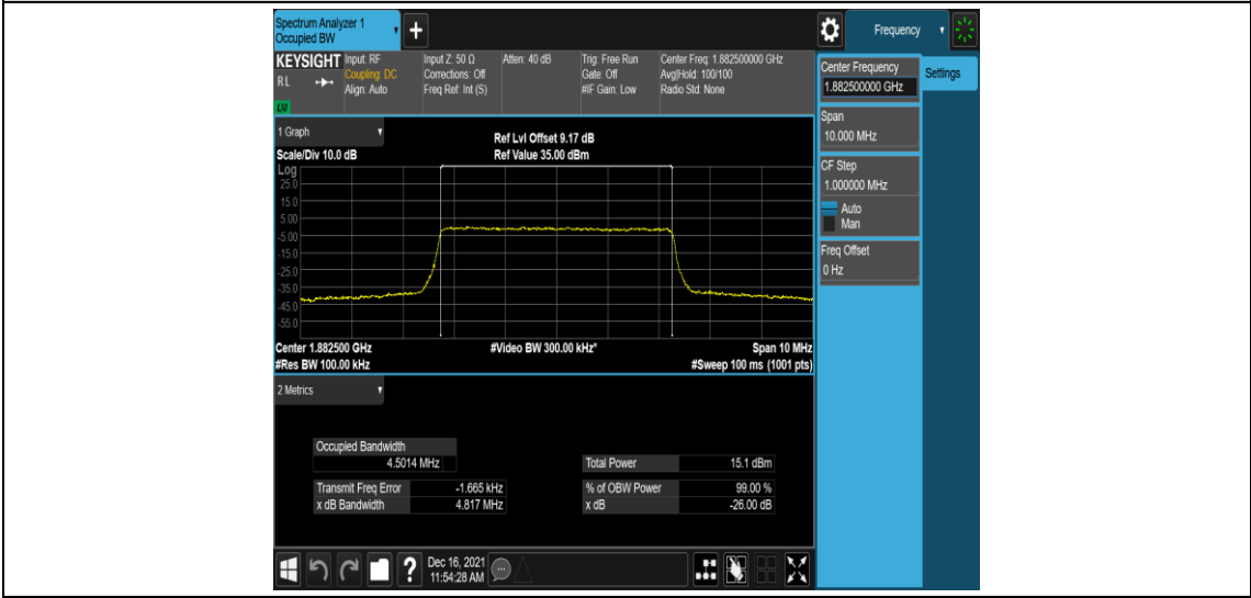
Band25-5MHz-QPSK-26365-25RB#0
