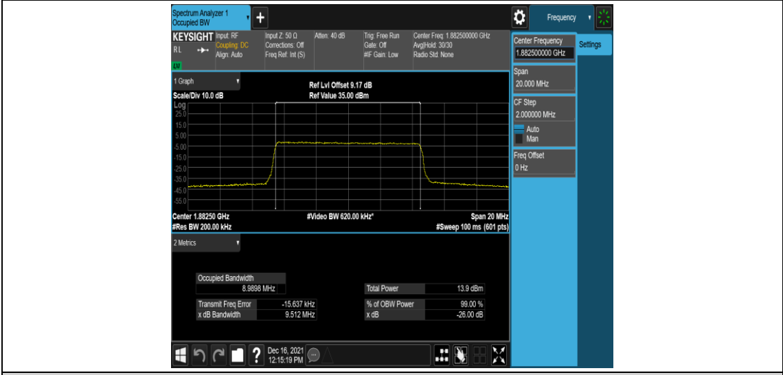
Band25-10MHz-QPSK-26365-50RB#0
