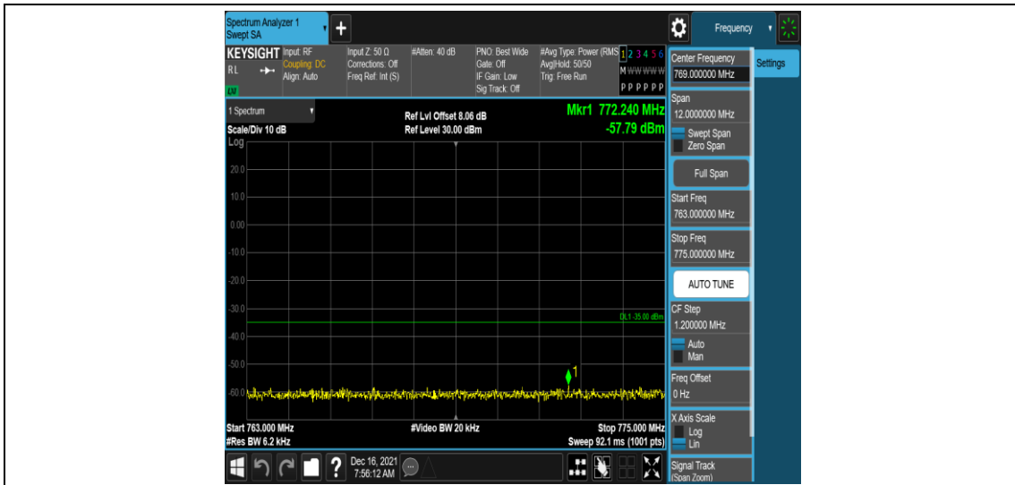
Band13-5MHz-16QAM-23230-1RB#0-Range5:763~775MHz
