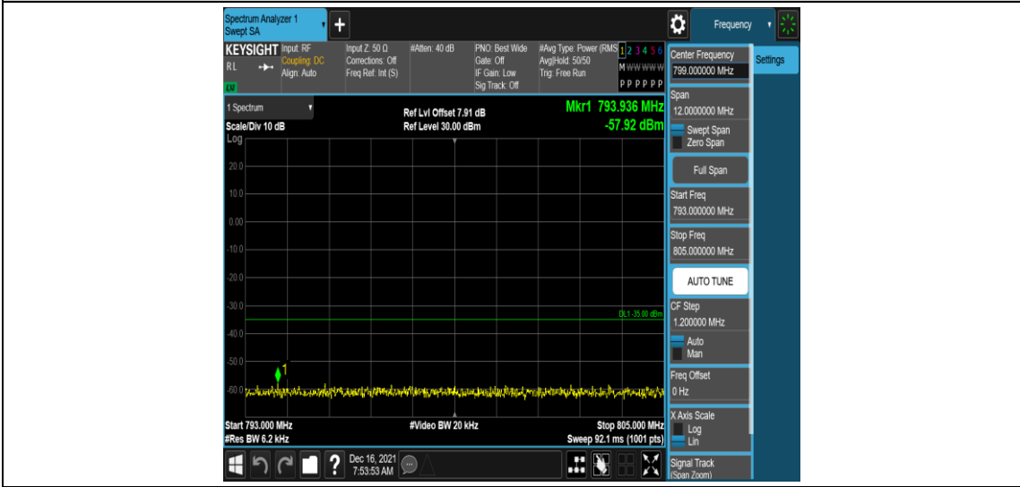
Band13-5MHz-QPSK-23230-1RB#0-Range6:793~805MHz
