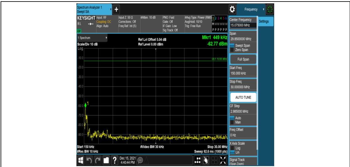
Band4-15MHz-QPSK-20025-1RB#0-Range2:0.15~30MHz
