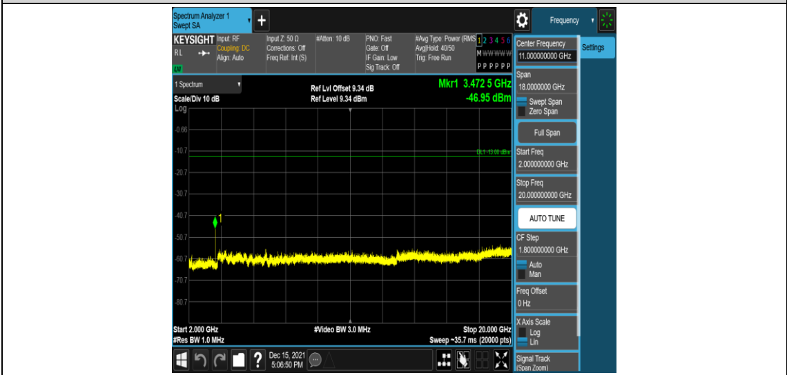
Band4-20MHz-QPSK-20300-1RB#0-Range5:2000~20000MHz
