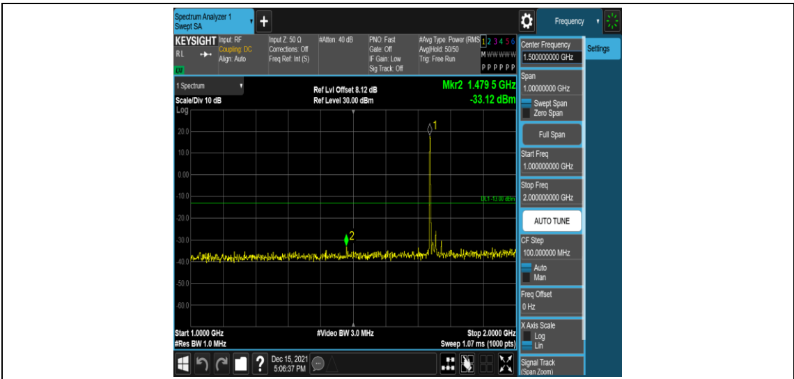
Band4-20MHz-QPSK-20300-1RB#0-Range4:1000~2000MHz
