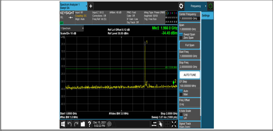
Band4-20MHz-QPSK-20050-1RB#0-Range4:1000~2000MHz
