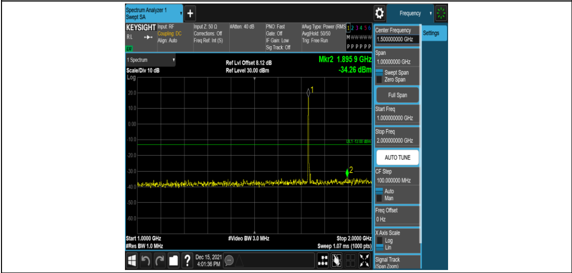
Band4-5MHz-QPSK-20175-1RB#0-Range4:1000~2000MHz
