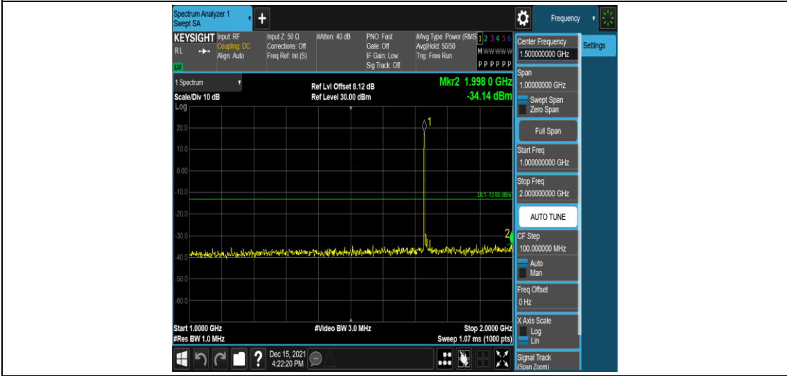
Band4-10MHz-QPSK-20175-1RB#0-Range4:1000~2000MHz
