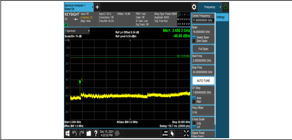
Band4-10MHz-QPSK-20175-1RB#0-Range5:2000~20000MHz
