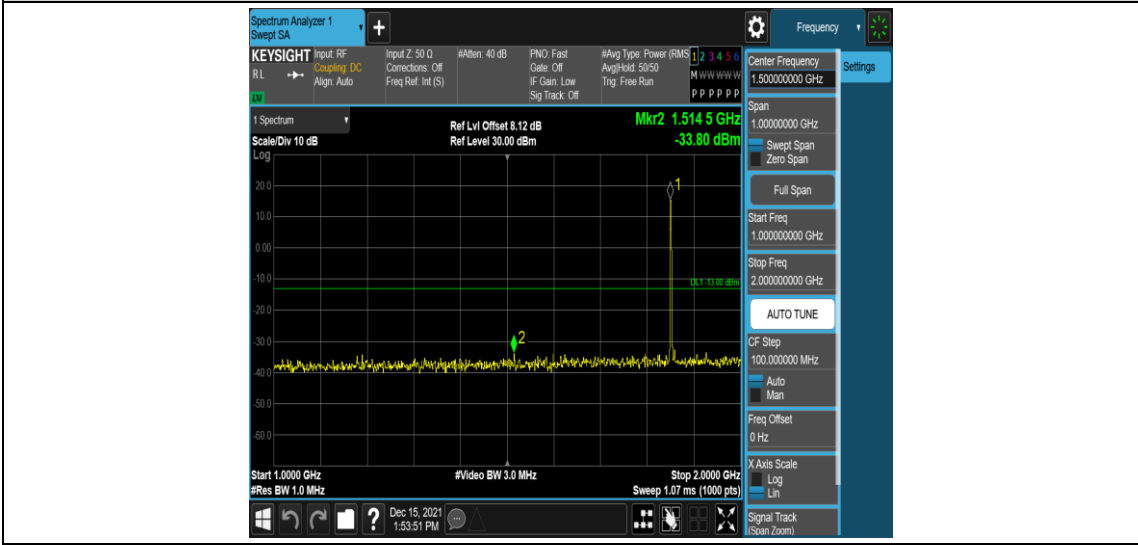
Band2-5MHz-QPSK-18625-1RB#0-Range4:1000~2000MHz
