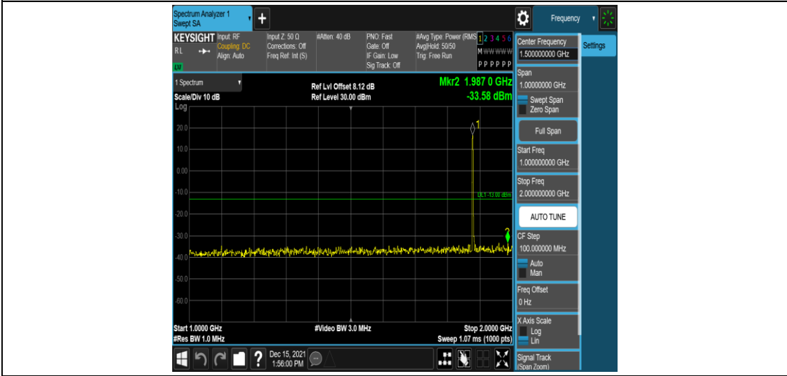
Band2-5MHz-QPSK-18900-1RB#0-Range4:1000~2000MHz
