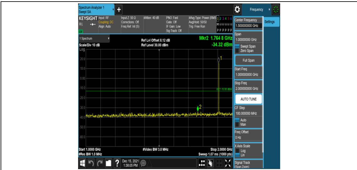
Band2-3MHz-16QAM-19185-1RB#0-Range4:1000~2000MHz
