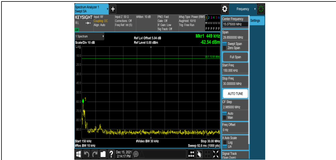
Band2-10MHz-QPSK-18650-1RB#0-Range2:0.15~30MHz
