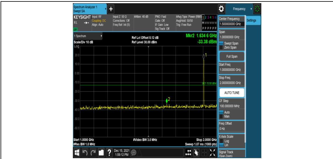
Band2-5MHz-16QAM-19175-1RB#0-Range4:1000~2000MHz
