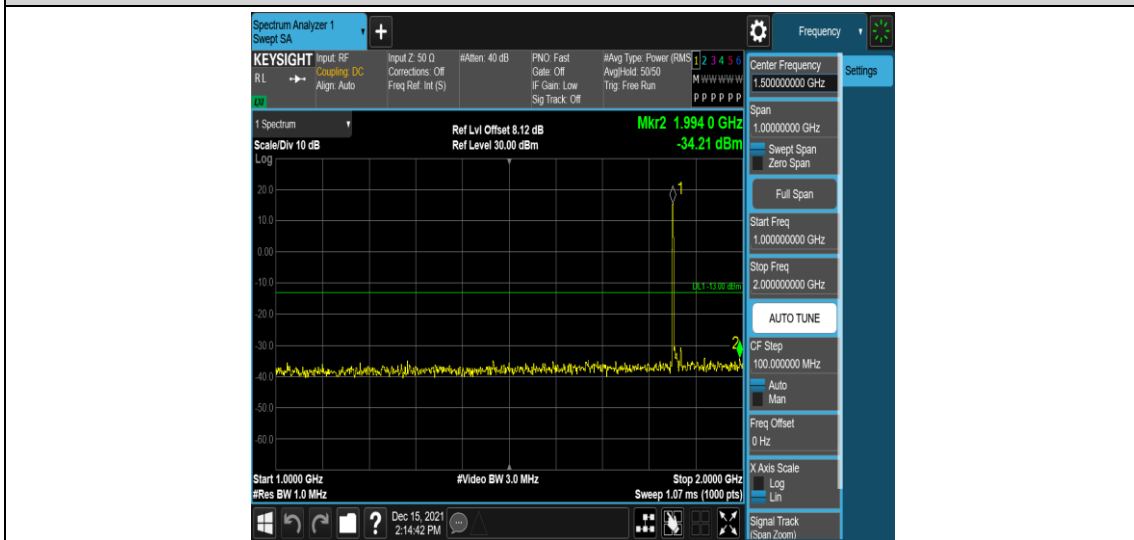
Band2-10MHz-QPSK-18650-1RB#0-Range4:1000~2000MHz
