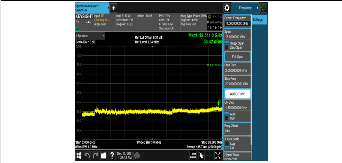
Band2-3MHz-QPSK-19185-1RB#0-Range5:2000~20000MHz
