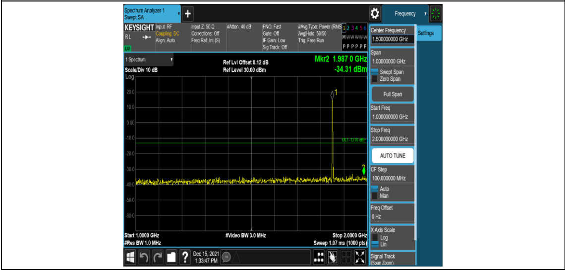
Band2-3MHz-16QAM-18615-1RB#0-Range4:1000~2000MHz
