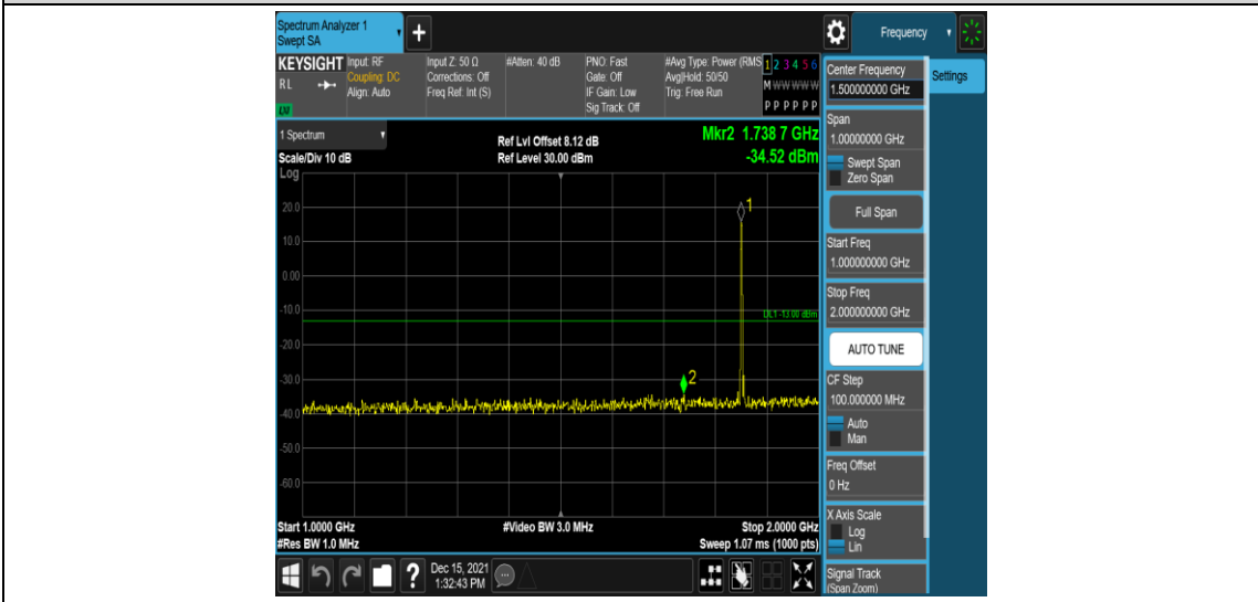
Band2-3MHz-QPSK-18615-1RB#0-Range4:1000~2000MHz
