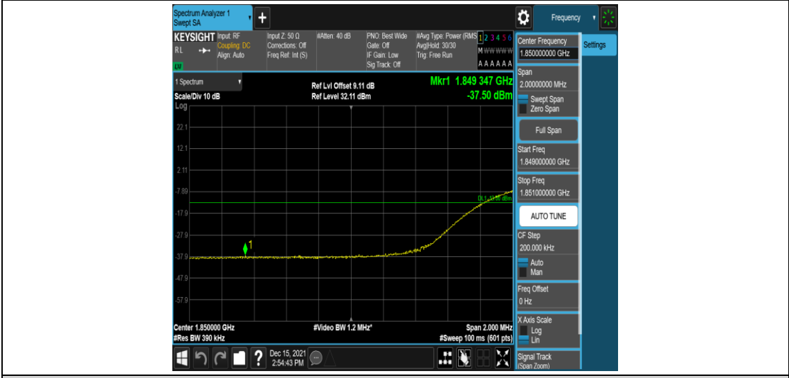
Band2-20MHz-16QAM-18700-100RB#0
