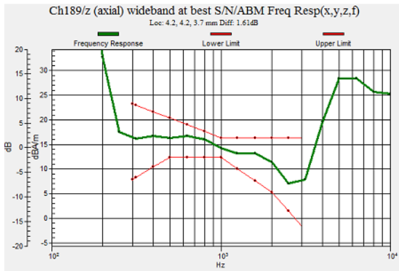
Fig 7.1 GSM850 Ch189
