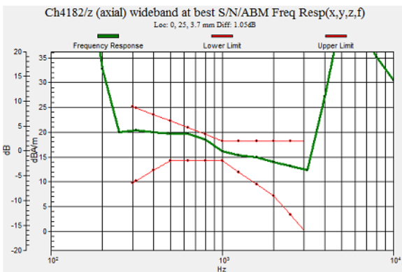
Fig 7.3 WCDMA Band V Ch4182
