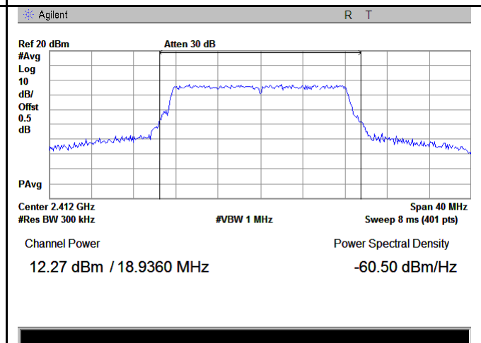
802.11g - AV Output power - Low CH 2412
