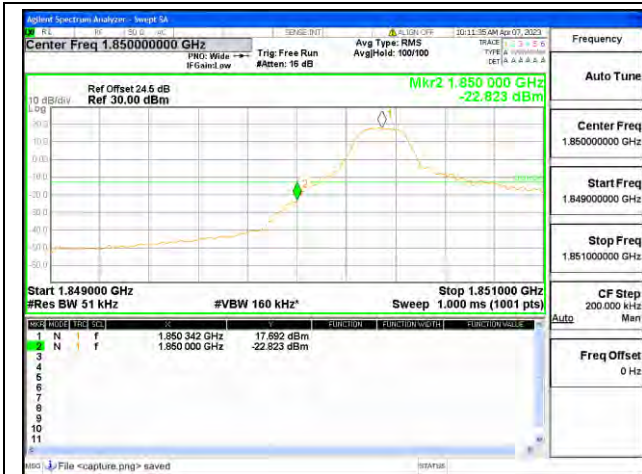
Band2 / 5MHz / Low CH / QPSK / 1 RB
