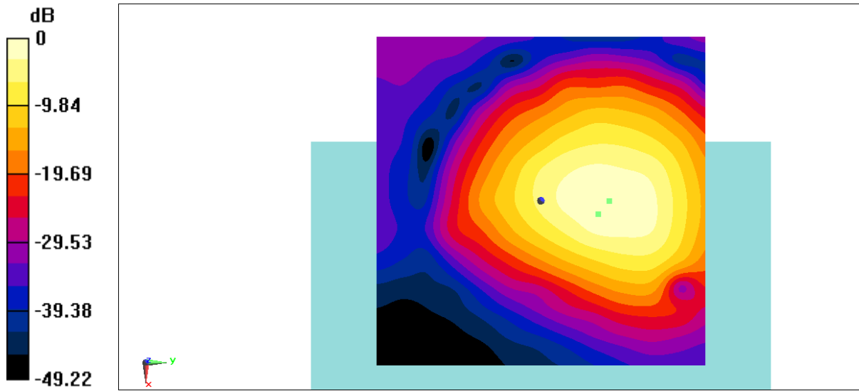
Fig B.4 T-Coil EDGE 1900
