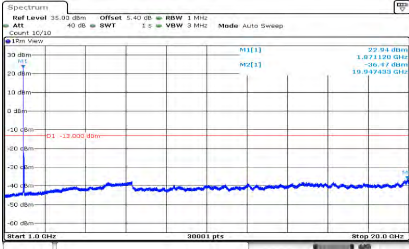
Band2-20MHz-16QAM-18900-1RB#0-Range2:1000~20000MHz
