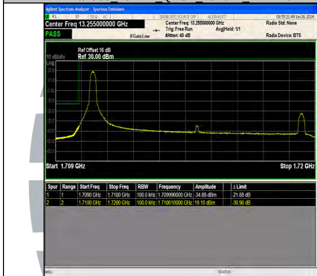
Band66 10MHz 64QAM 132022 1RB#0
