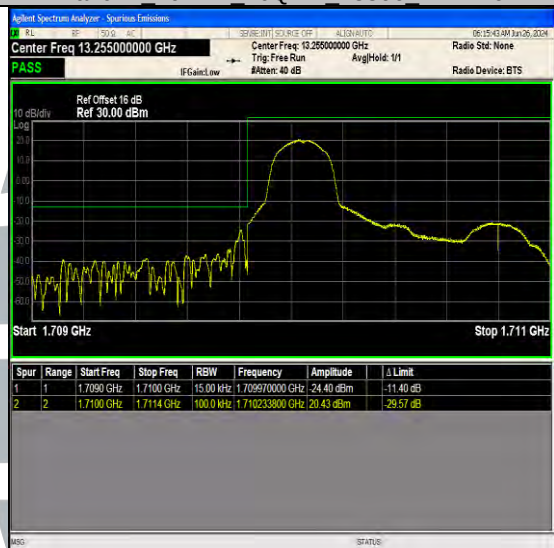
Band66 1.4MHz QPSK 131979 1RB#0
