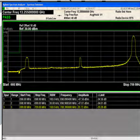
Band12 10MHz QPSK 23060 1RB#49
