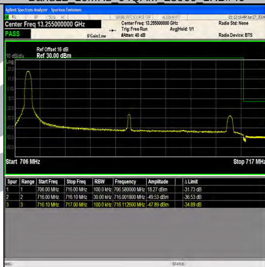
Band12 10MHz 64QAM 23130 1RB#0
