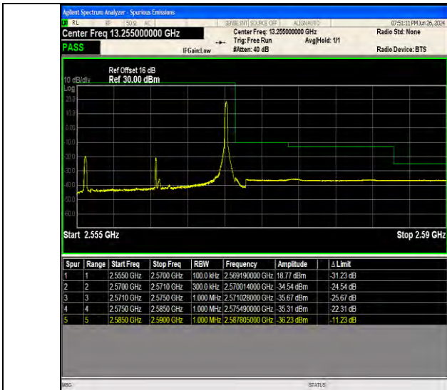
Band7 15MHz QPSK 21375 1RB#74
