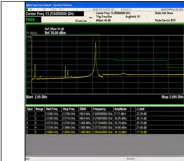
Band7 20MHz 64QAM 21350 1RB#99
