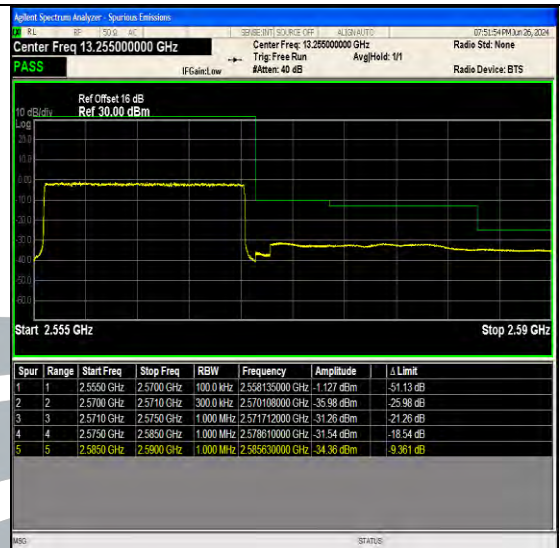
Band7 15MHz QPSK 21375 75RB#0
