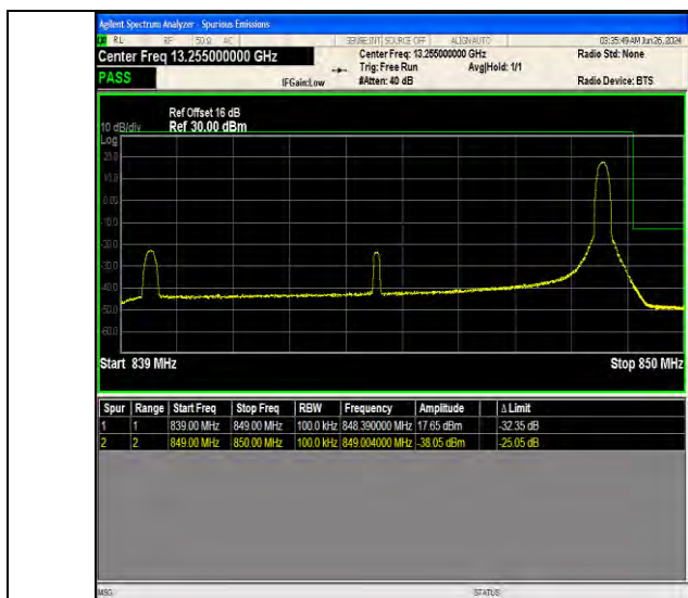
Band5 10MHz 64QAM 20600 1RB#49
