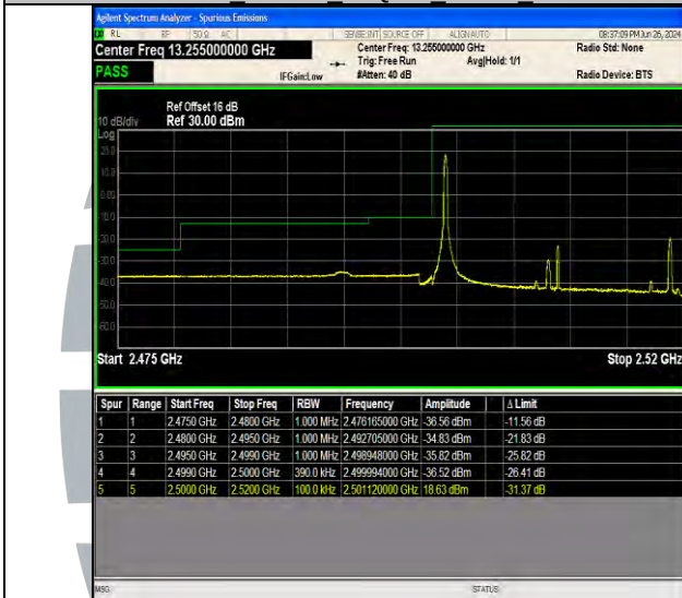
Band7 20MHz QPSK 20850 1RB#0
