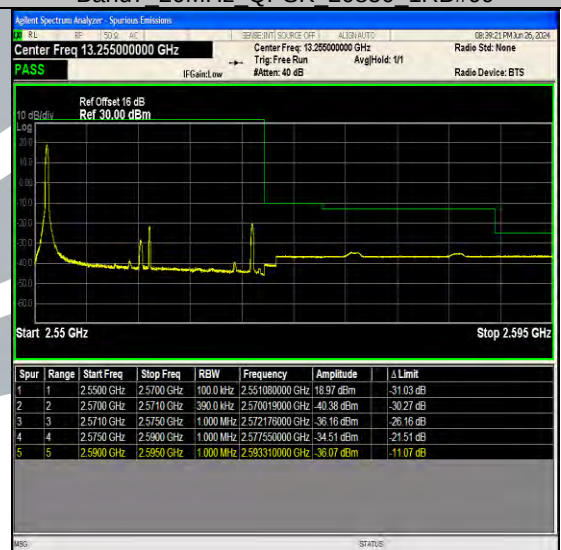
Band7 20MHz QPSK 21350 1RB#0
