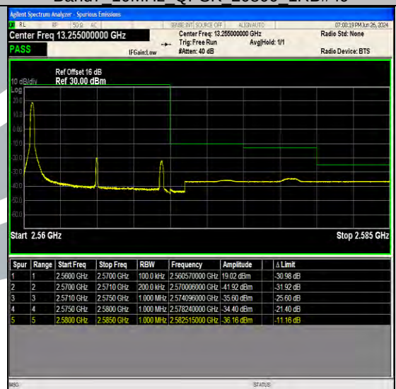
Band7 10MHz QPSK 21400 1RB#0
