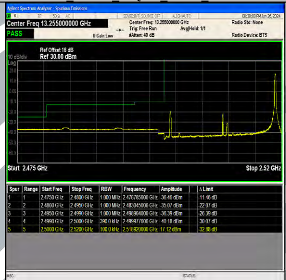
Band7 20MHz 16QAM 20850 1RB#99
