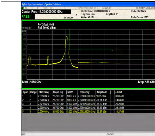
Band7 5MHz 64QAM 21425 1RB#24
