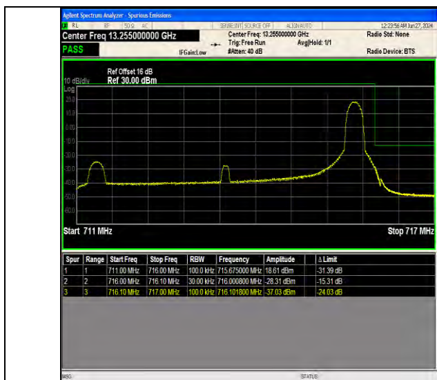
Band12 5MHz 64QAM 23155 1RB#24
