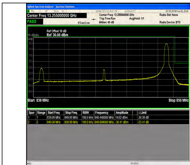
Band5 10MHz QPSK 20600 1RB#49
