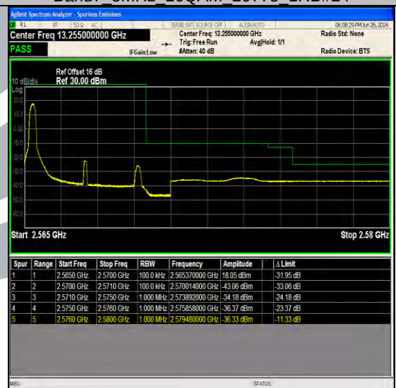
Band7 5MHz 16QAM 21425 1RB#0
