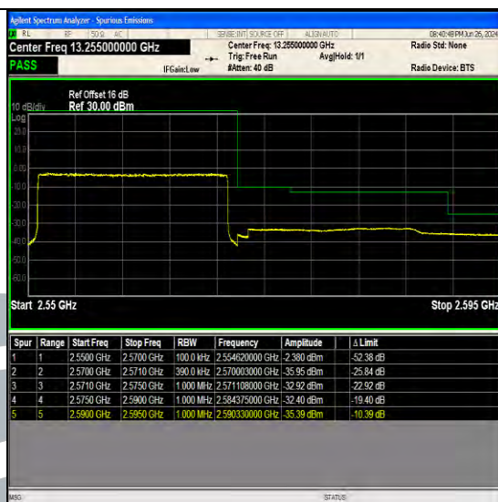
Band7 20MHz QPSK 21350 100RB#0
