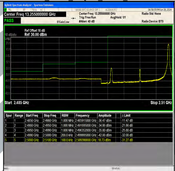
Band7 10MHz QPSK 20800 1RB#49
