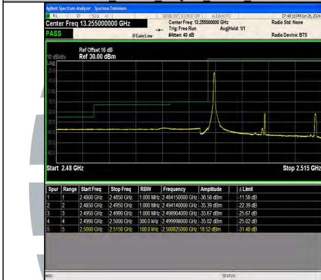
Band7 15MHz QPSK 20825 1RB#0
