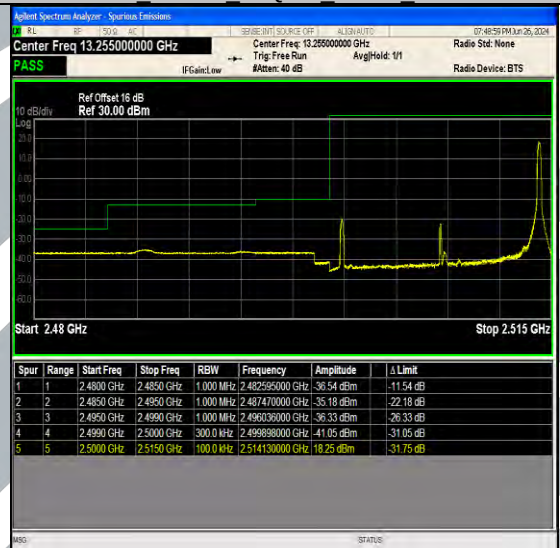
Band7 15MHz QPSK 20825 1RB#74
