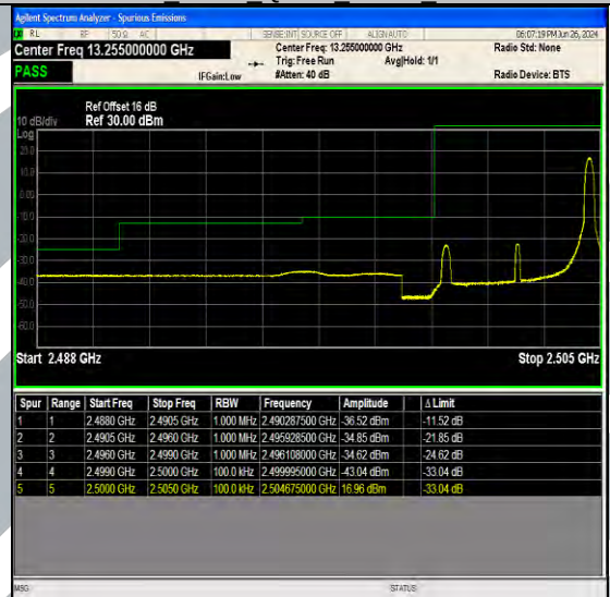
Band7 5MHz 64QAM 20775 1RB#24
