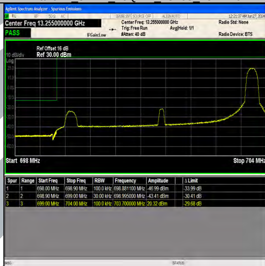
Band12 5MHz QPSK 23035 1RB#24
