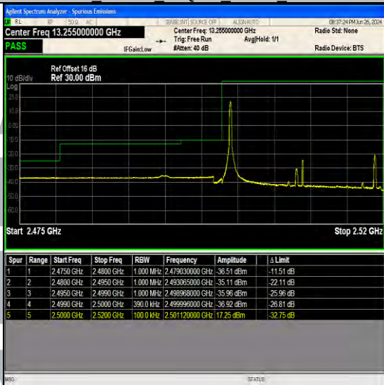
Band7 20MHz 16QAM 20850 1RB#0
