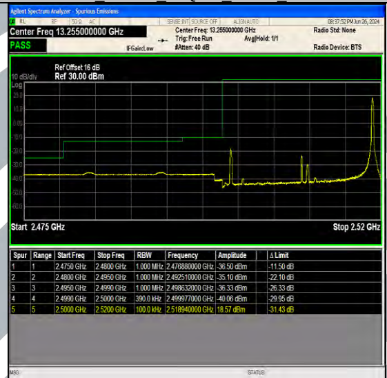
Band7 20MHz QPSK 20850 1RB#99
