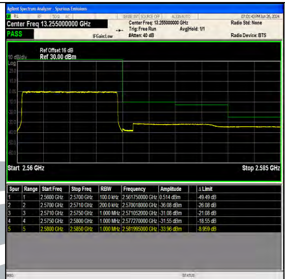
Band7 10MHz QPSK 21400 50RB#0
