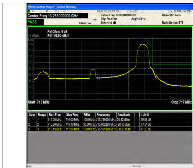
Band12 3MHz QPSK 23165 1RB#14
