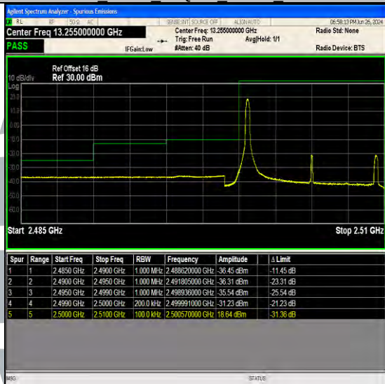
Band7 10MHz QPSK 20800 1RB#0
