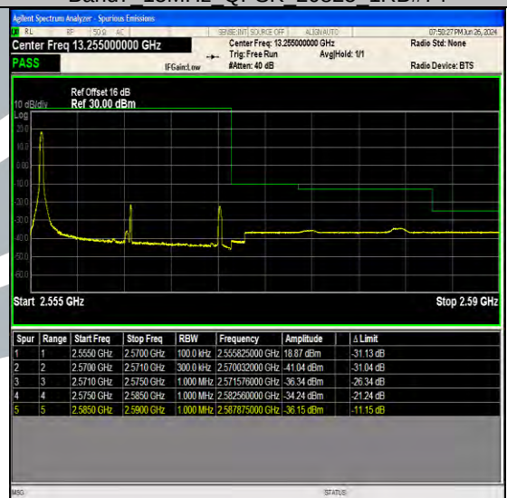
Band7 15MHz QPSK 21375 1RB#0
