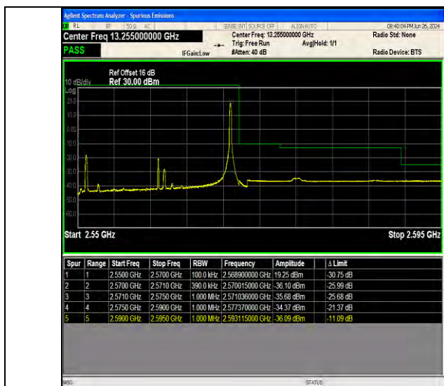
Band7 20MHz QPSK 21350 1RB#99
