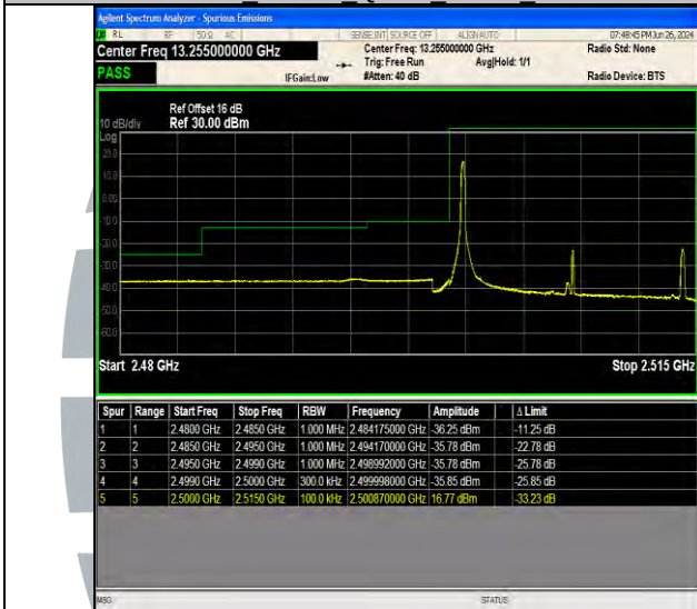
Band7 15MHz 64QAM 20825 1RB#0
