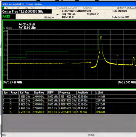
Band7 5MHz 64QAM 20775 1RB#0
