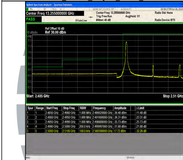
Band7 10MHz 16QAM 20800 1RB#0
