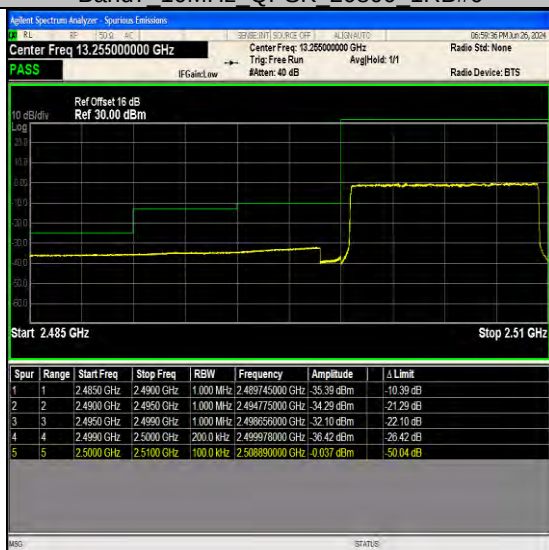
Band7 10MHz QPSK 20800 50RB#0
