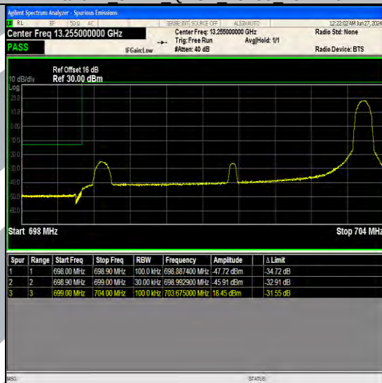
Band12 5MHz 64QAM 23035 1RB#24
