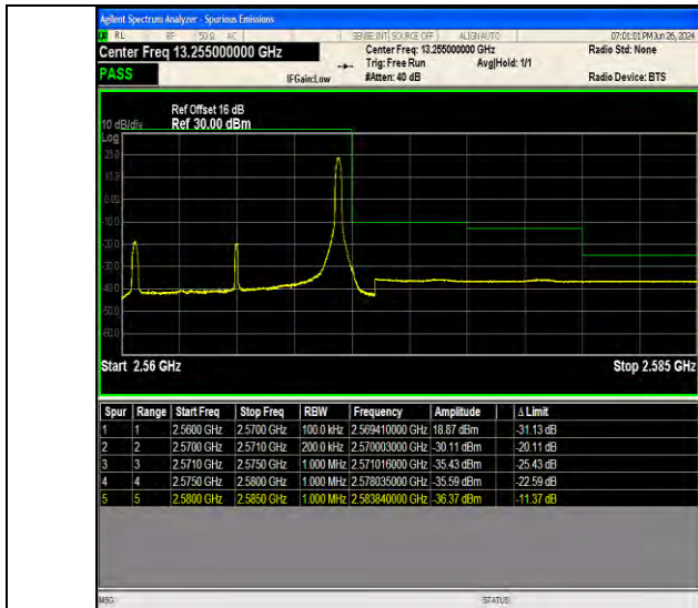
Band7 10MHz QPSK 21400 1RB#49
