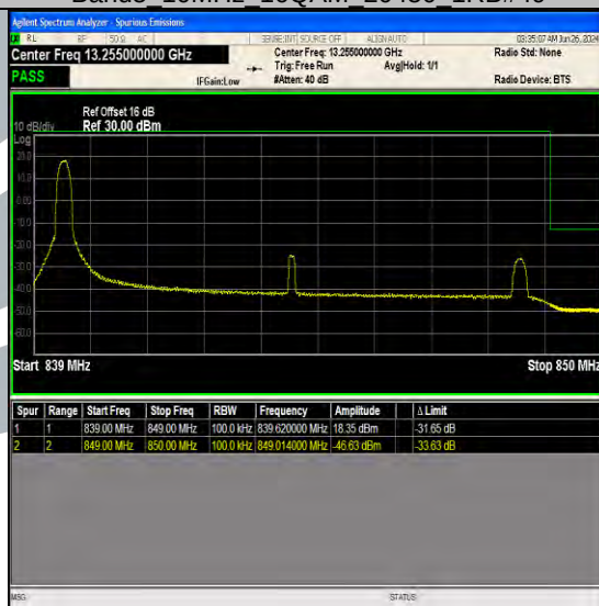
Band5 10MHz 16QAM 20600 1RB#0
