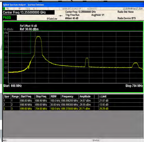
Band12 5MHz QPSK 23035 1RB#0
