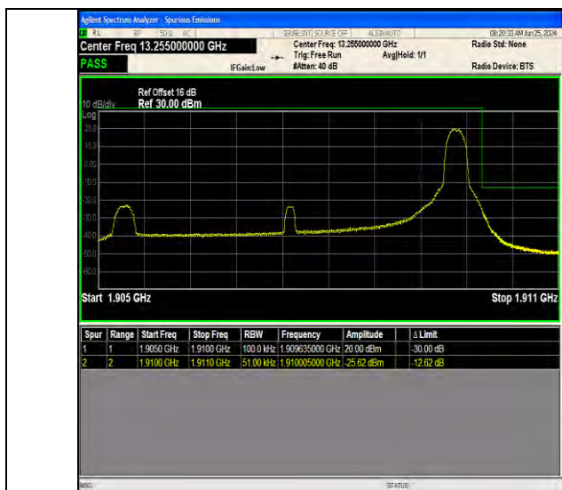
Band2 5MHz QPSK 19175 1RB#24
