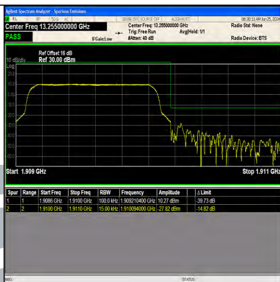
Band2 1.4MHz QPSK 19193 6RB#0
