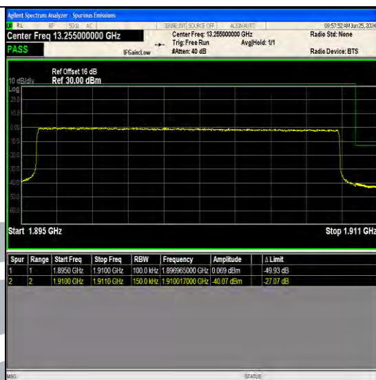
Band2 15MHz QPSK 19125 75RB#0
