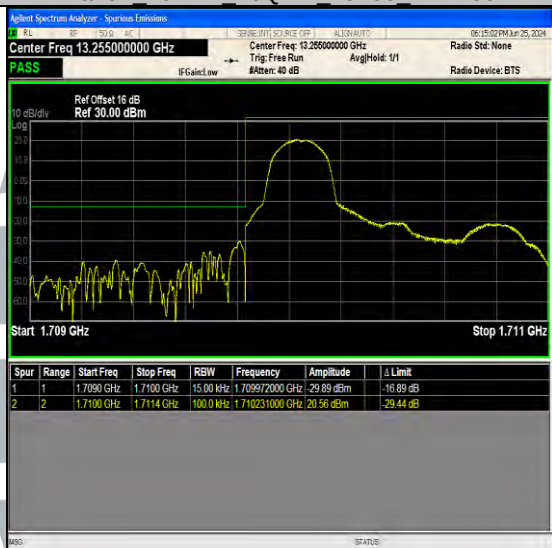
Band4 1.4MHz QPSK 19957 1RB#0
