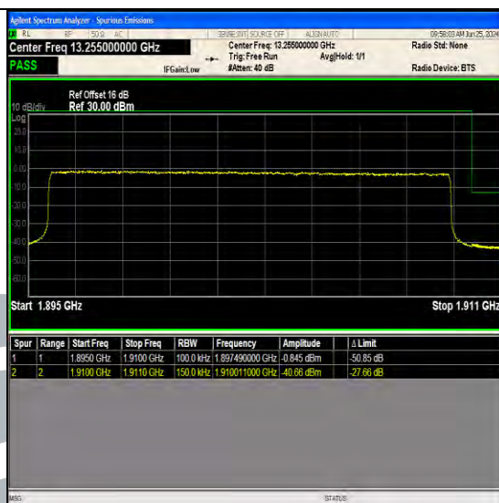
Band2 15MHz 16QAM 19125 75RB#0
