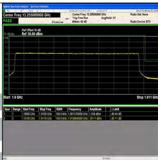
Band2 10MHz QPSK 19150 50RB#0
