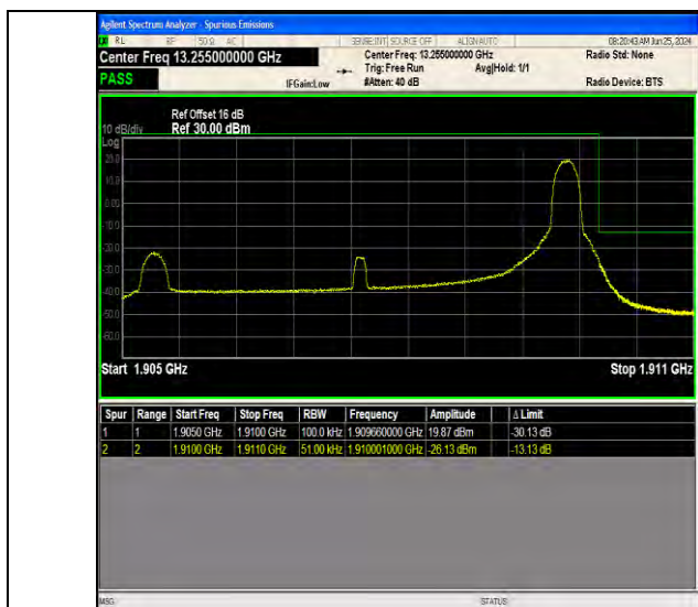
Band2 5MHz 16QAM 19175 1RB#24
