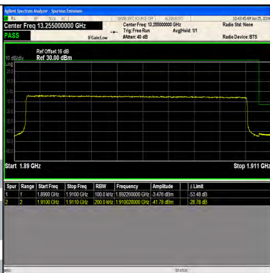
Band2 20MHz 64QAM 19100 100RB#0
