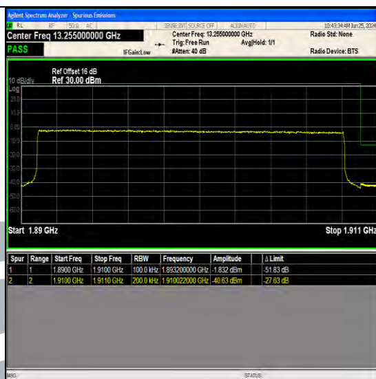
Band2 20MHz 16QAM 19100 100RB#0
