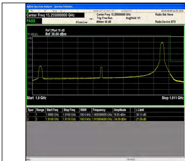
Band2 10MHz QPSK 19150 1RB#49
