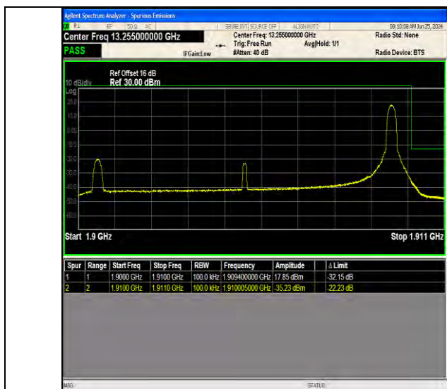
Band2 10MHz 64QAM 19150 1RB#49
