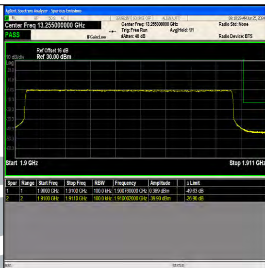
Band2 10MHz 16QAM 19150 50RB#0
