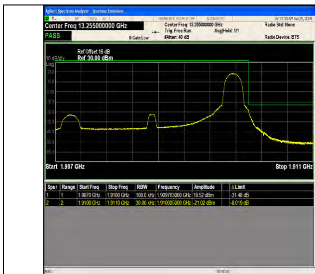
Band2 3MHz 64QAM 19185 1RB#14
