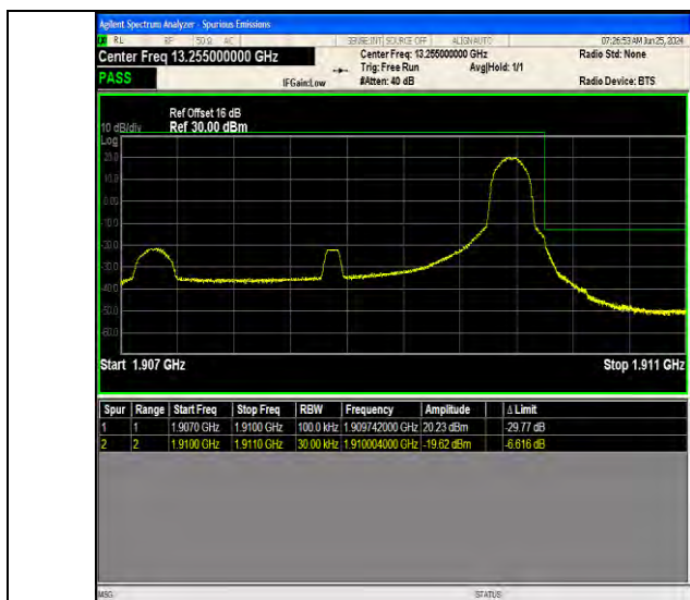
Band2 3MHz QPSK 19185 1RB#14
