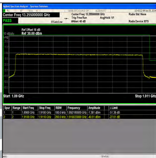
Band2 20MHz QPSK 19100 100RB#0
