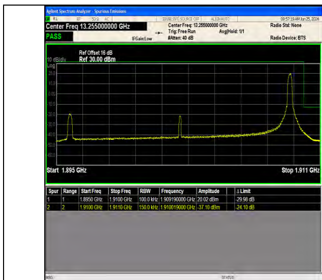
Band2 15MHz QPSK 19125 1RB#74
