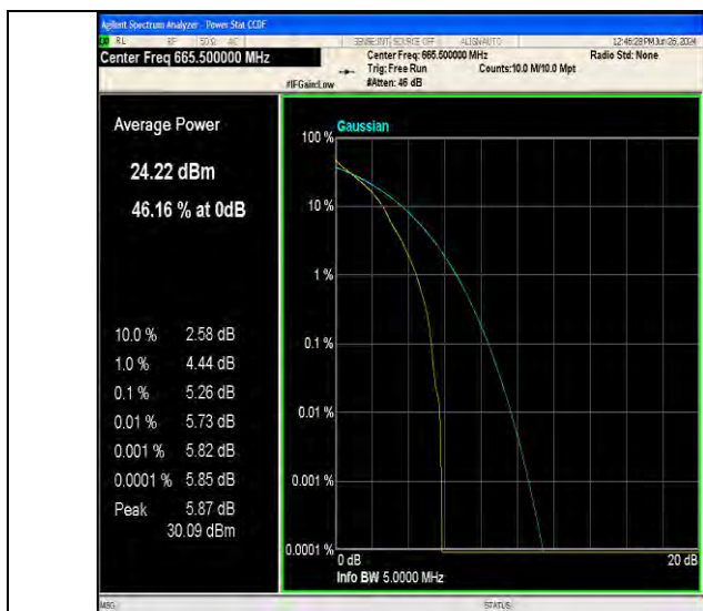
Band71-5MHz-QPSK-133147-1RB#0-PASS
