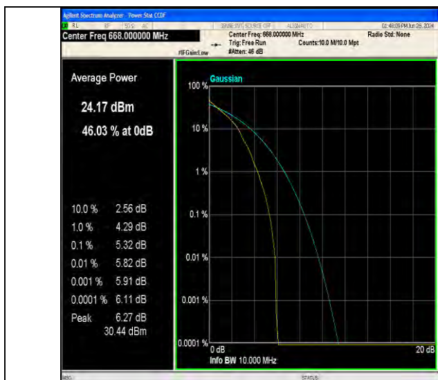
Band71-10MHz-QPSK-133172-1RB#0-PASS
