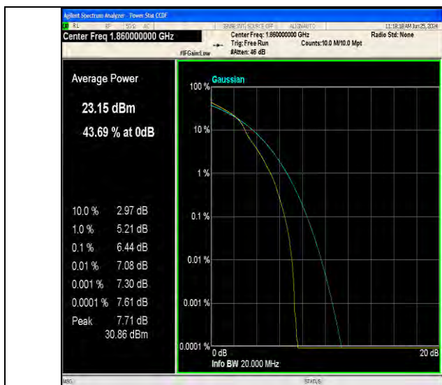
Band2-20MHz-16QAM-18700-1RB#0-PASS
