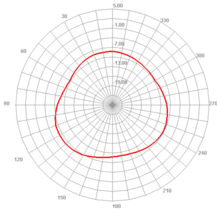
5150.000MHz E2
