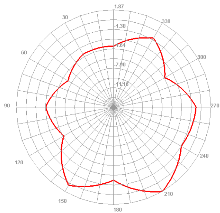
2450.000MHz E2
