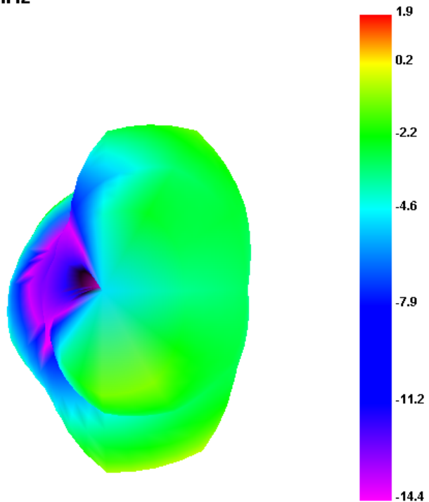
2450.000MHz E1
