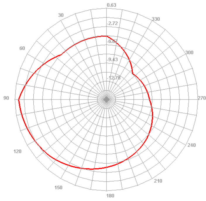
1820.000MHz E2
