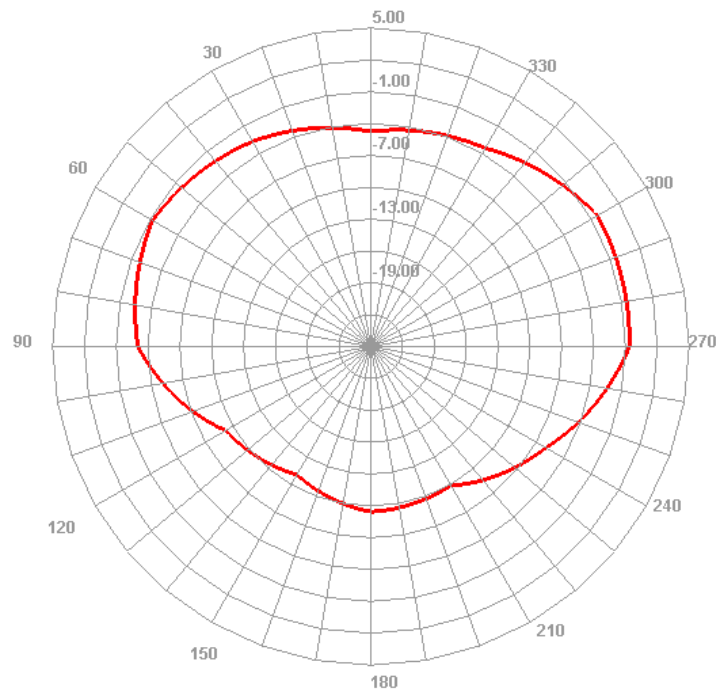
2450.000MHz E2
