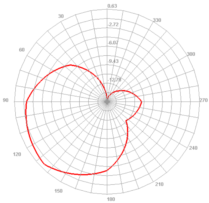
1820.000MHz E1
